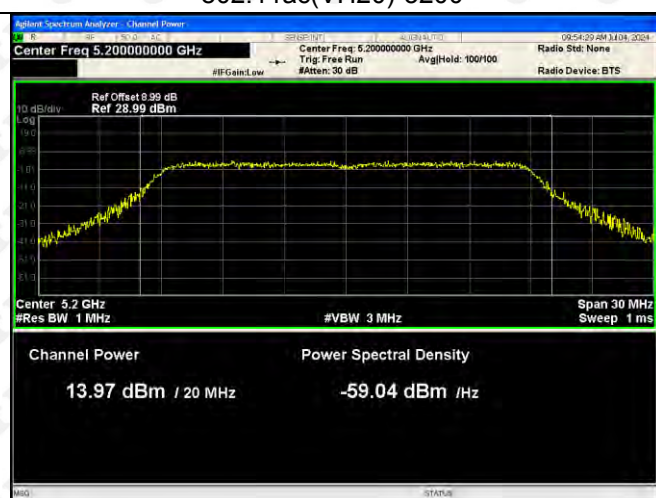
802.11ac(VH20)-5200
