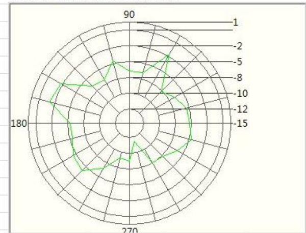
2.5GHz E2
