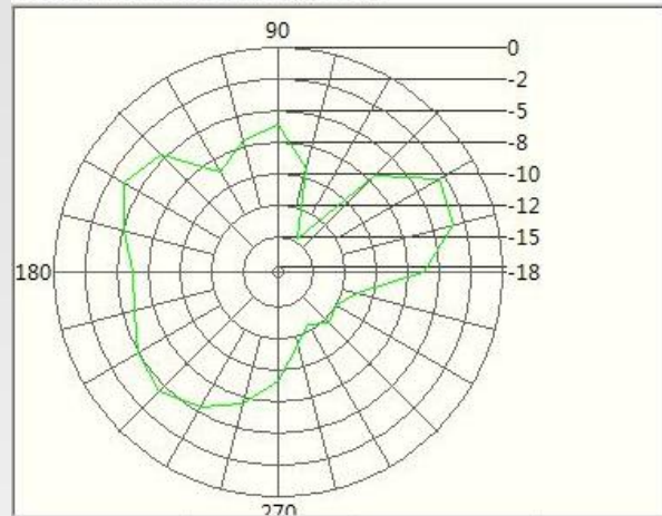
2.5GHz H
