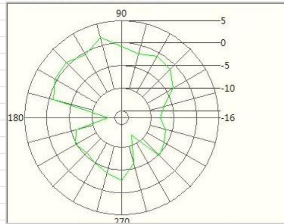
2.5GHz E1
