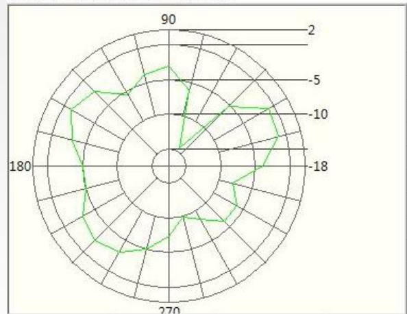
2.5GHz H
