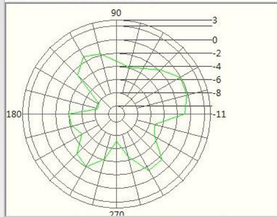
2.5GHz H
