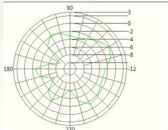
2.5GHz H
