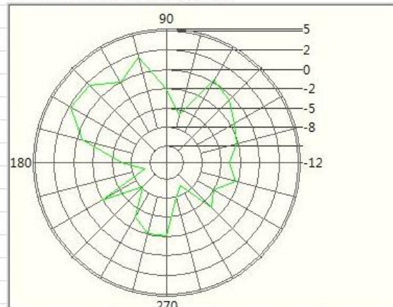
2.5GHz E1
