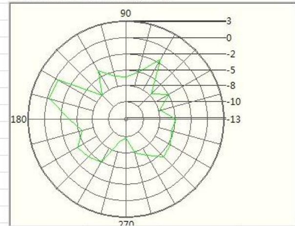
2.5GHz E2
