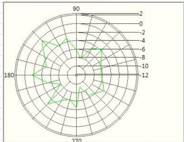
2.5GHz E1
