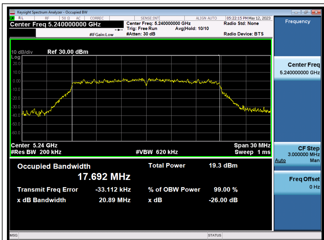
802.11ac20_ANT1_5240_MCS0_OBW
