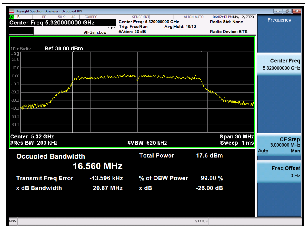
802.11a_ANT1_5320_6Mbps_OBW
