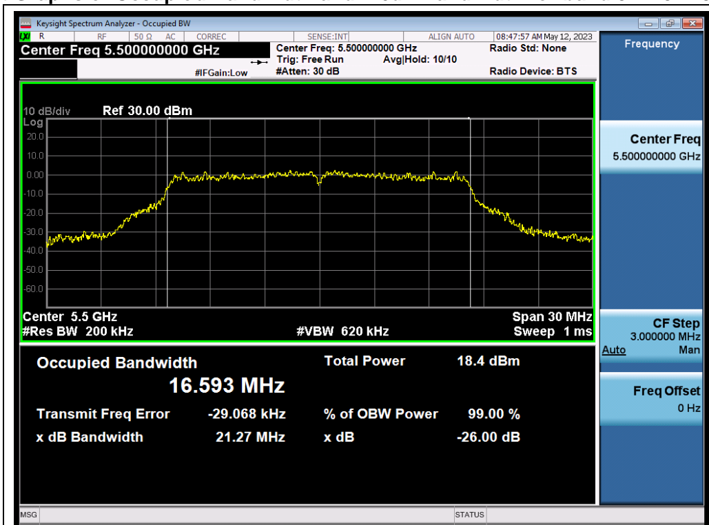
802.11a_ANT1_5500_6Mbps_OBW
