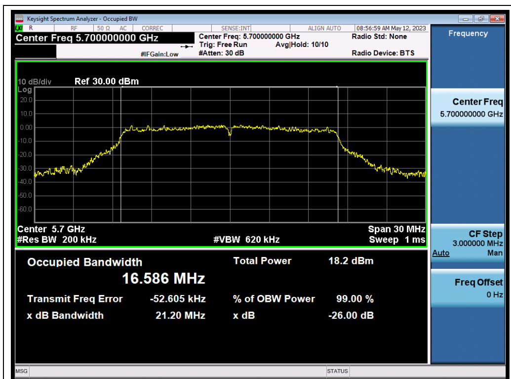
802.11a_ANT1_5700_6Mbps_OBW
