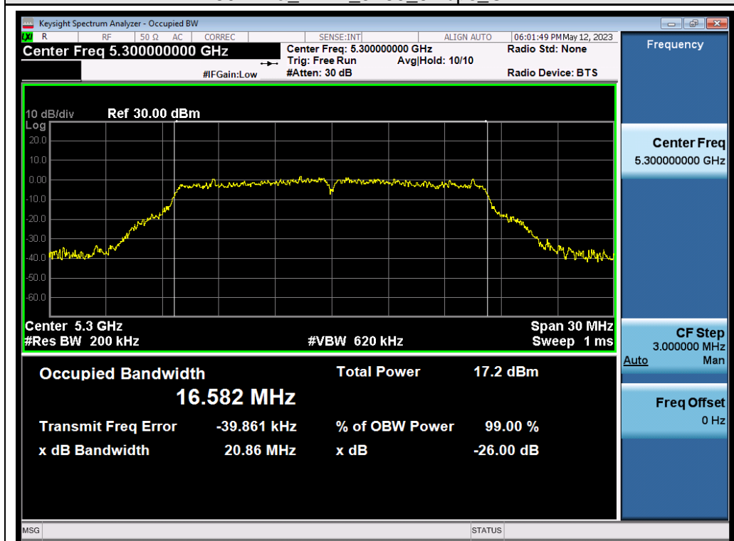
802.11a_ANT1_5300_6Mbps_OBW
