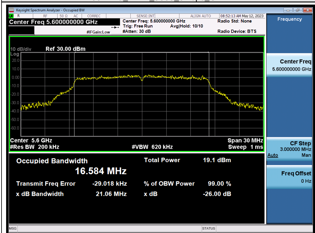
802.11a_ANT1_5600_6Mbps_OBW
