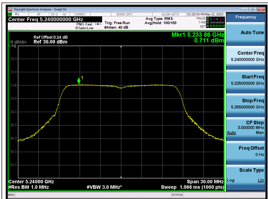
802.11a ANT1 5240 6Mbps PSD
