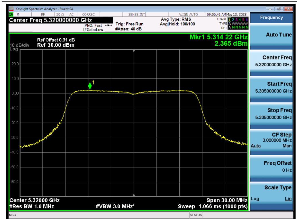
802.11a ANT1 5320 6Mbps PSD
