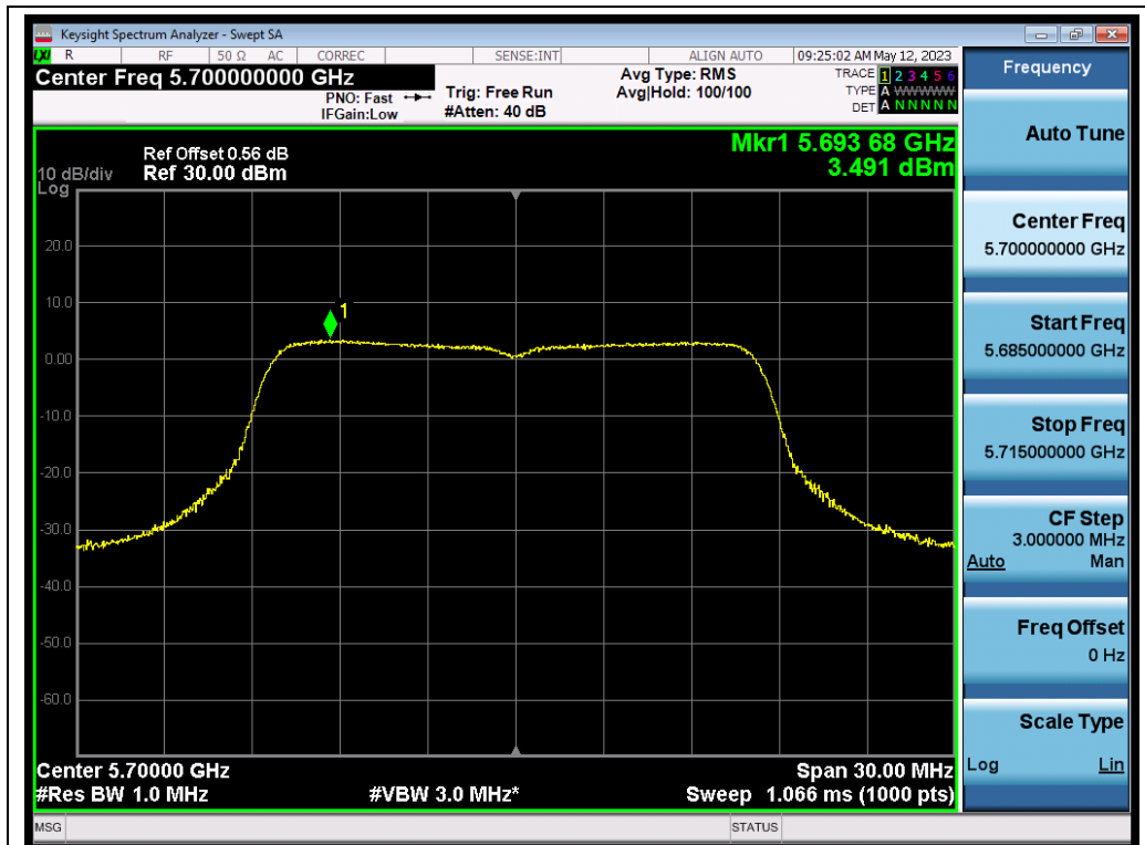
802.11a ANT1 5700 6Mbps PSD
