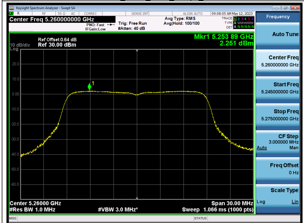
802.11n20 ANT1 5260 MCS0 PSD
