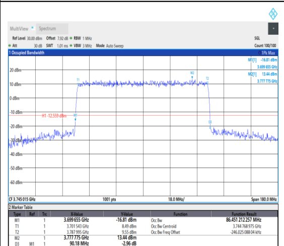
1-N77-3700-3980--30-90-L-4-DFT-64QAM-O
