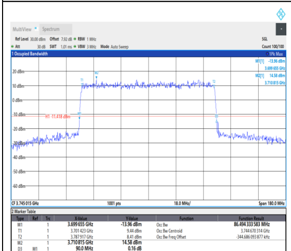
1-N77-3700-3980--30-90-L-3-DFT-16QAM-O
