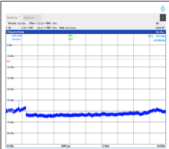
1-N78-3450-3550--30-100-L-1-DFT-PI2BPSK -Inner_1RB_Left-1@1-6000-18000-Ant1-697 4.88--54.72--13-
