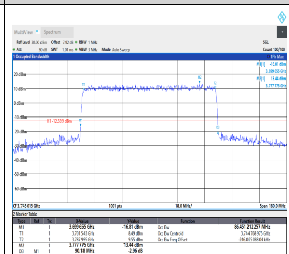
1-N77-3700-3980--30-90-L-4-DFT-64QAM-O
