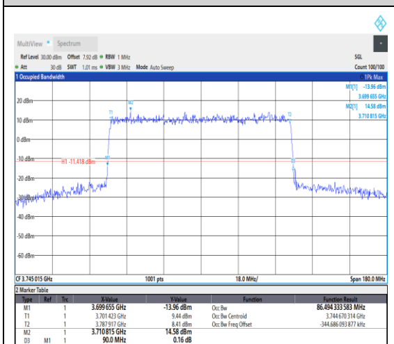
1-N77-3700-3980--30-90-L-3-DFT-16QAM-O
