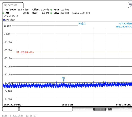
11G-Ant1-2462-30~1000-PASS
