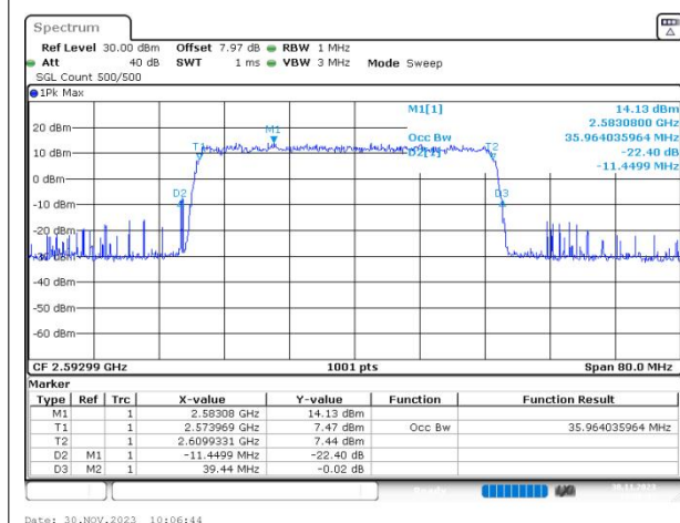
n41 SCS=30kHz DFT_BPSK BW=40MHz Channel=518598 RB=100@0
