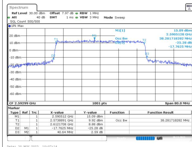
n41 SCS=30kHz CP_16QAM BW=40MHz Channel=518598 RB=106@0
