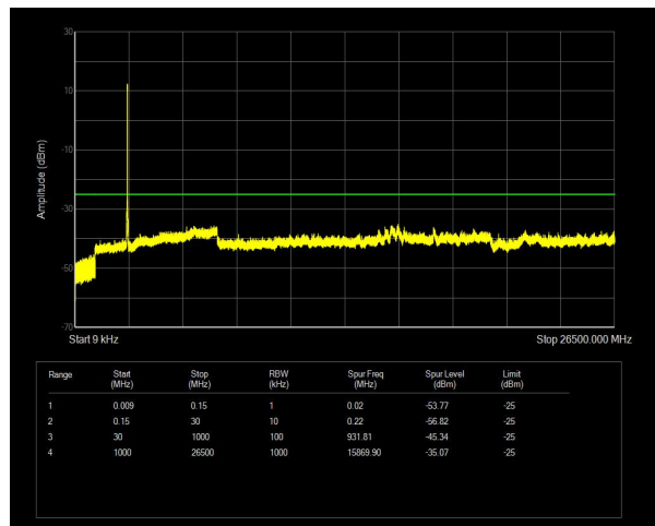
n38 SCS=30kHz DFT_BPSK BW=20MHz Channel=516000 RB=50@0
