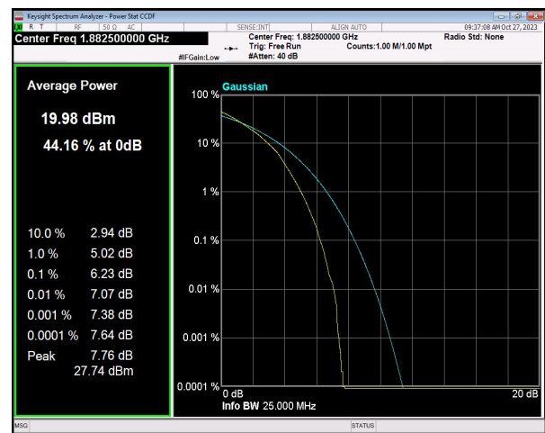
n25 SCS=15kHz DFT_QAM64 BW=20MHz Channel=376500 RB=100@0
