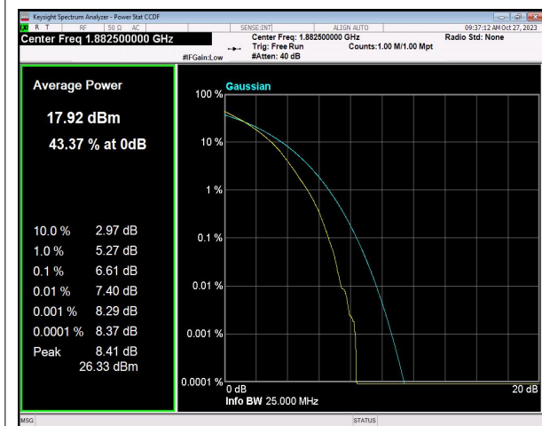
n25 SCS=15kHz DFT_QAM256 BW=20MHz Channel=376500 RB=100@0
