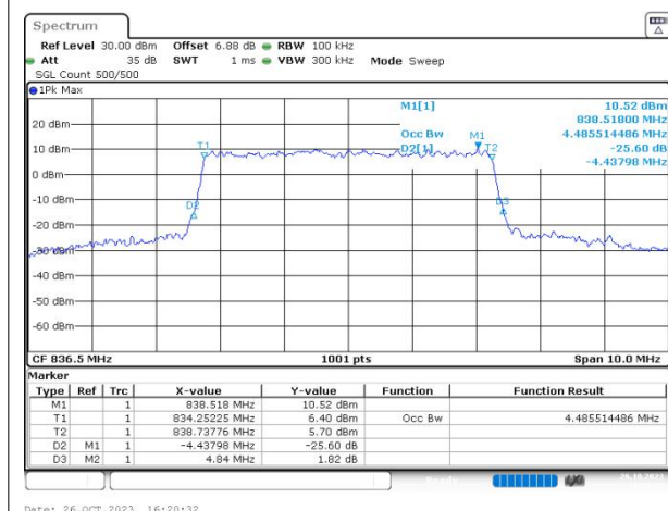
n5 SCS=15kHz CP_QAM256 BW=5MHz Channel=167300 RB=25@0
