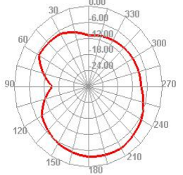
2410.000MHz H
