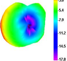
2450.000MHz
