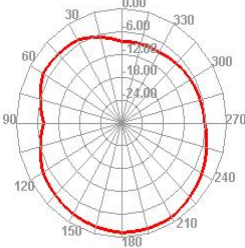
2450.000MHz H
