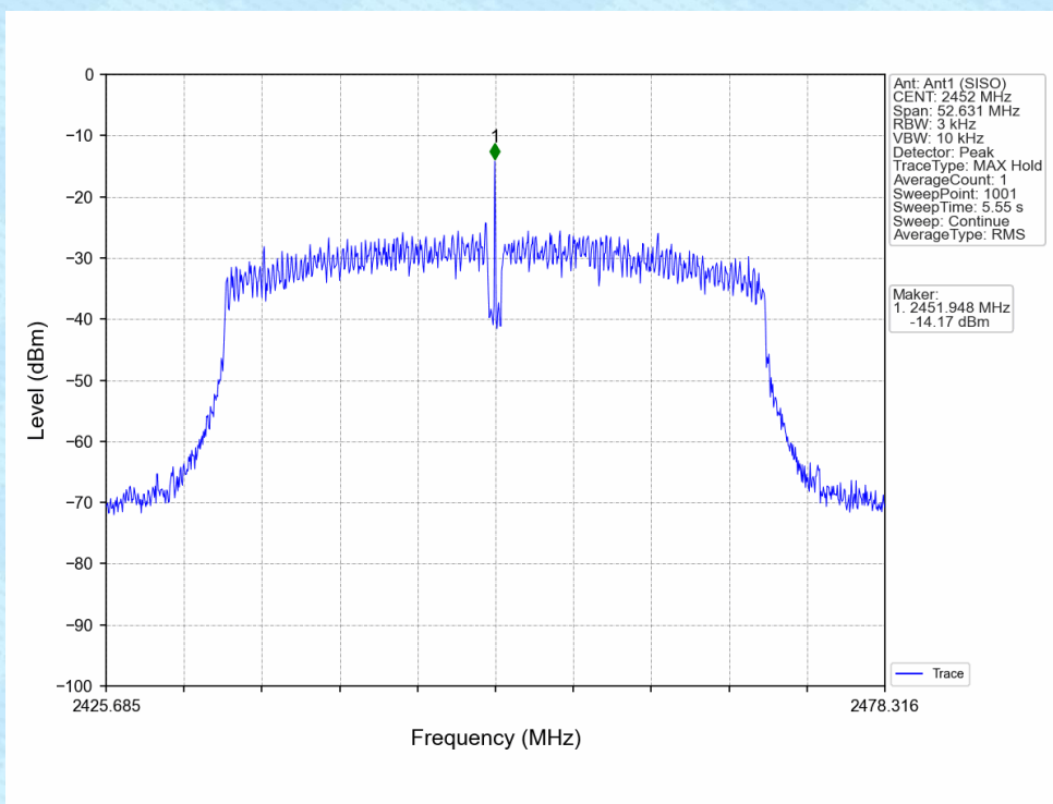
802.11n(HT40)_HCH_2452MHz_Ant1 (SISO)_NTNV
