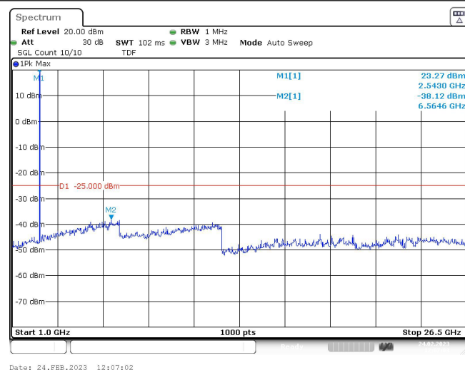
Band41-5MHz-QPSK-40265-1RB#0-Range2:1000~26500MHz
