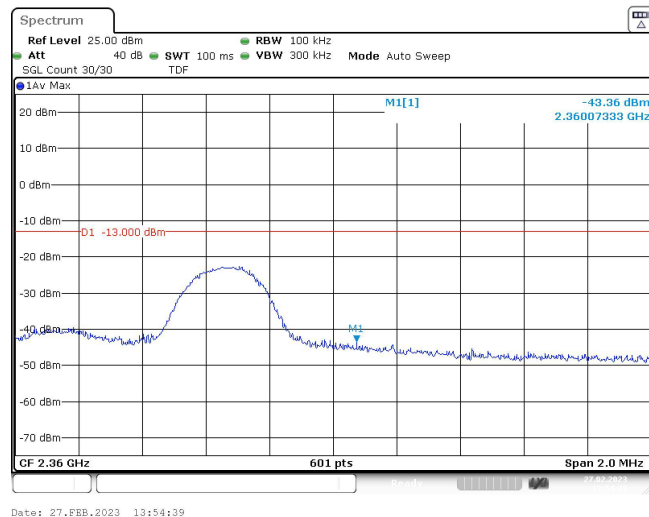
Band40-5MHz-QPSK-39225-1RB#24
