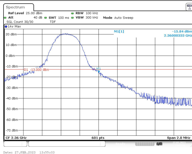
Band40-5MHz-QPSK-39225-25RB#0
