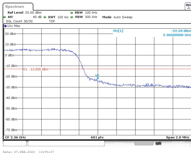
Band40-10MHz-QPSK-39200-1RB#0
