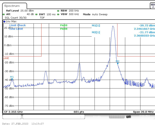
Band40-10MHz-QPSK-39200-50RB#0
