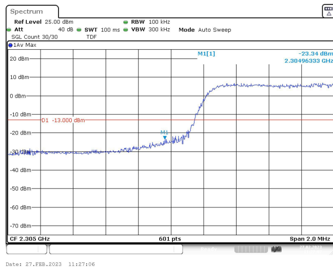
Band40-5MHz-QPSK-38775-1RB#0
