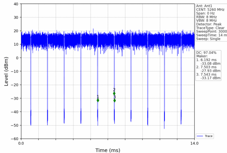
802.11n(HT20)_LCH_5260MHz_Ant1_NTNV
