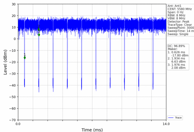
802.11n(HT20)_MCH_5580MHz_Ant1_NTNV
