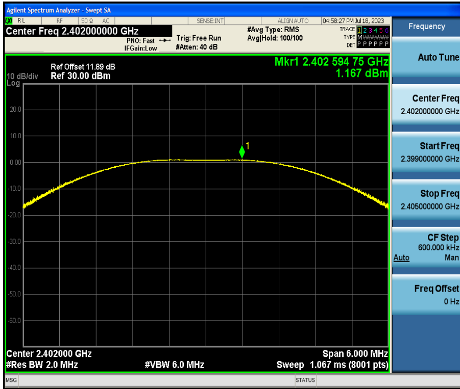
BLE_2M-Ant1-2402
