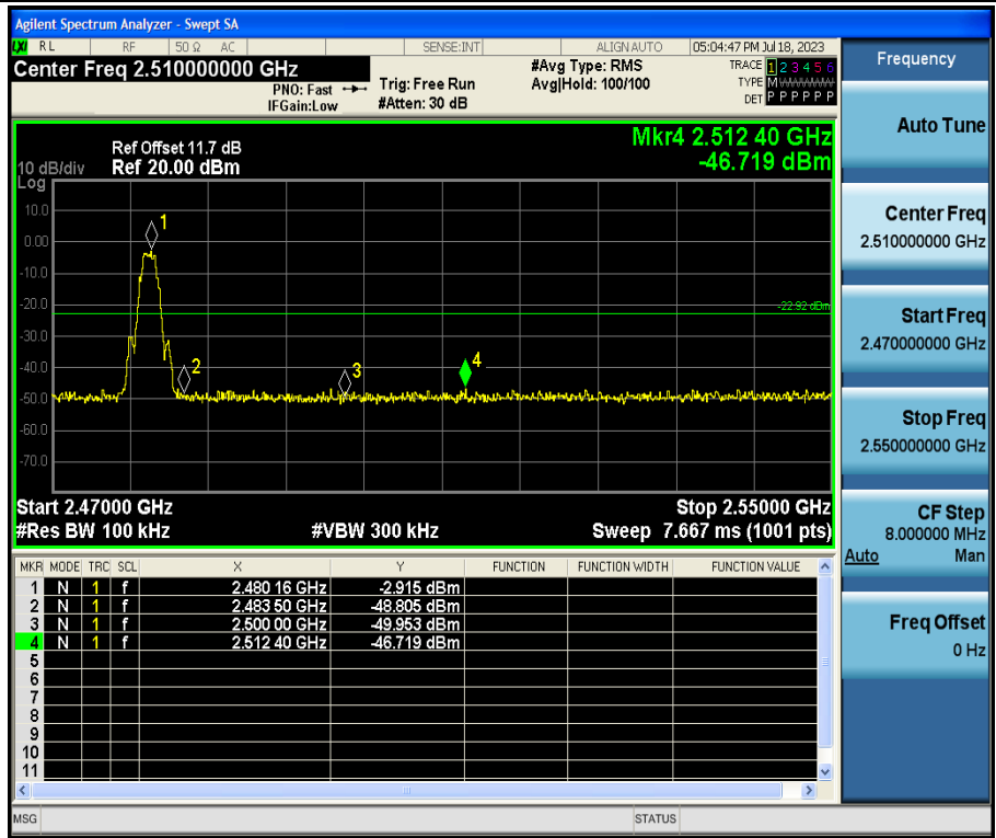
BLE_2M-Ant1-2480
