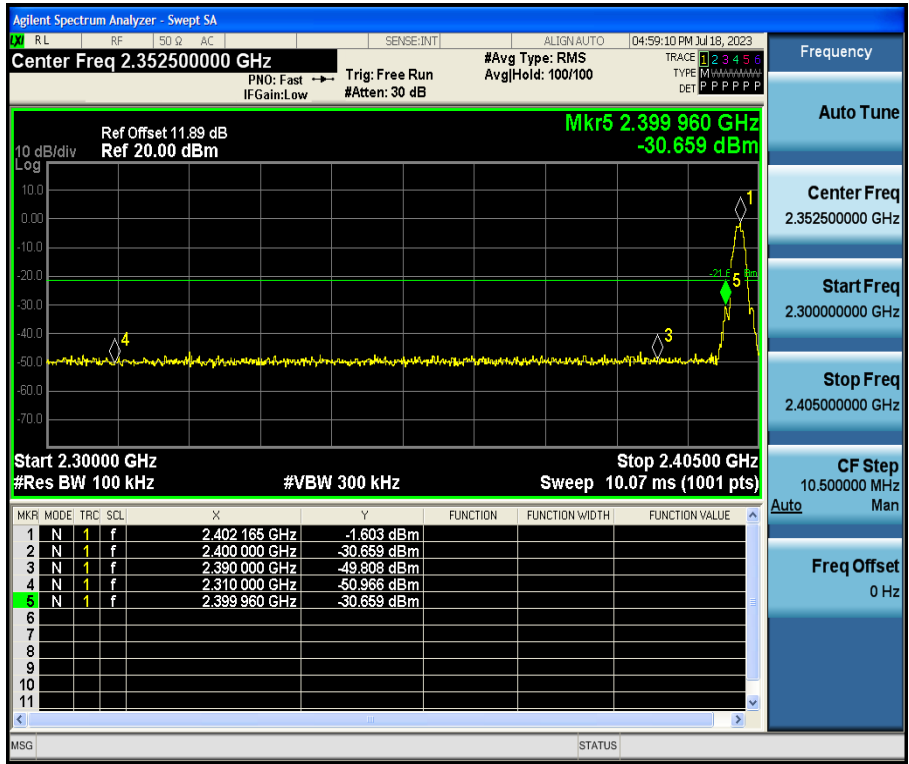
BLE_2M-Ant1-2402
