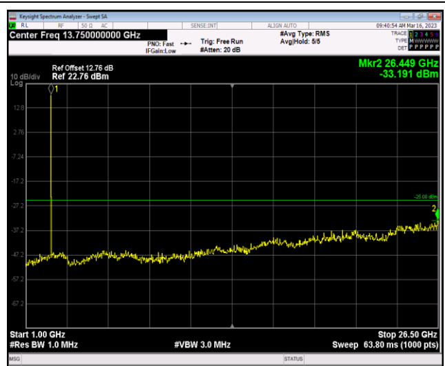
Band7-20MHz-QPSK-20850-1RB#0-Range2:1000~26500MHz
