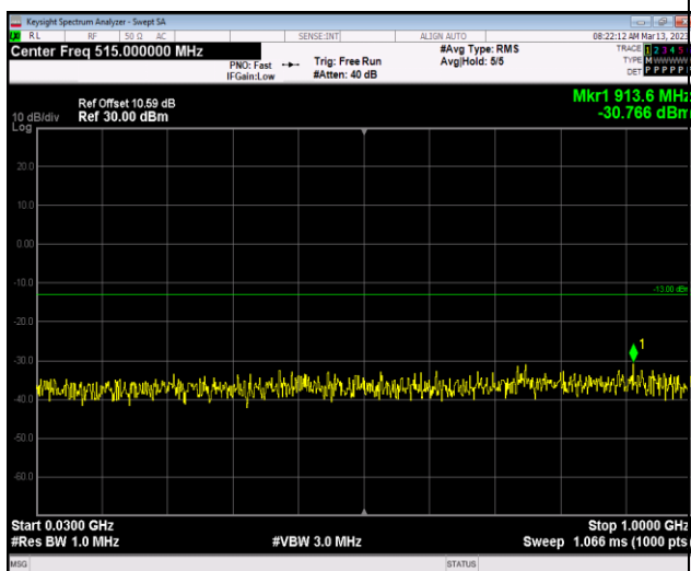
Band4-20MHz-QPSK-20050-1RB#0-Range1:30~1 000MHz
