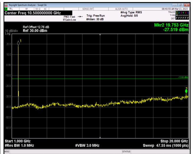
Band4-20MHz-QPSK-20300-1RB#0-Range2:1000~20000MHz
