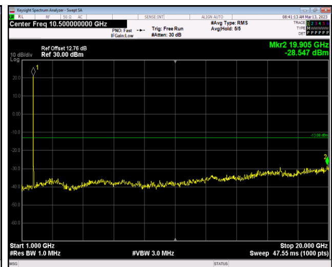
Band4-20MHz-16QAM-20300-1RB#0-Range2:1000~2 0000MHz
