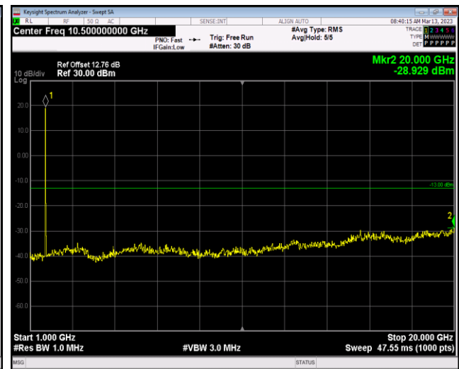
Band4-20MHz-16QAM-20175-1RB#0-Range2:1000~2 0000MHz
