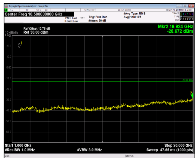
Band4-20MHz-QPSK-20050-1RB#0-Range2:1000~20 000MHz
