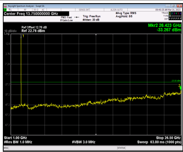
Band7-5MHz-16QAM-21425-1RB#0-Range2:1000~26 500MHz
