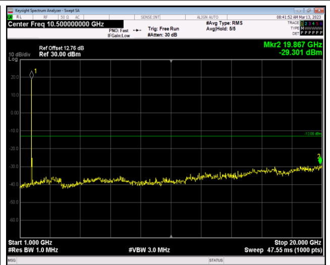
Band4-20MHz-QPSK-20300-1RB#0-Range2:1000~20000MHz
