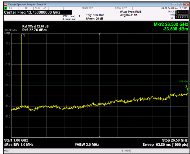
Band7-5MHz-16QAM-21425-1RB#0-Range2:1000~26 500MHz
