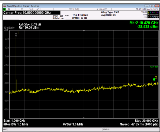
Band2-20MHz-16QAM-18900-1RB#0-Range2:1000~20000MHz
