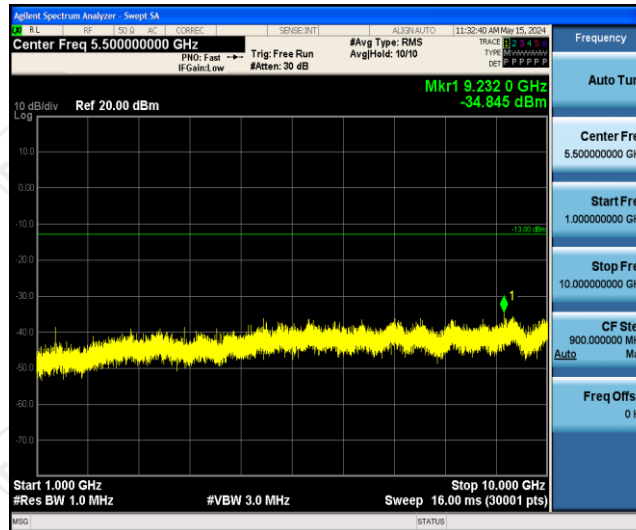
Band71-5MHz-QPSK-133147-1RB#0-Range2:1000~10000MHz
