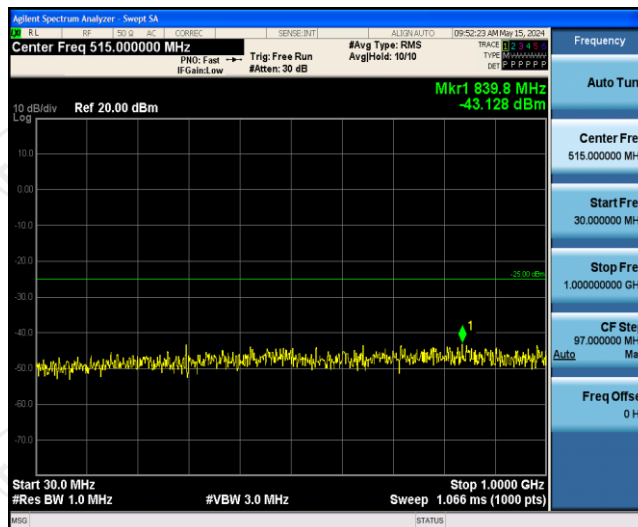
Band41-10MHz-QPSK-39700-1RB#0-Range1:30~1000MHz
