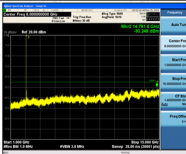
Band41-10MHz-QPSK-39700-1RB#0-Range2:1000~15000MHz
