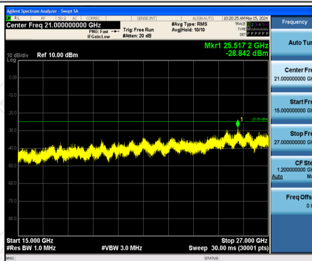
Band41-20MHz-QPSK-41490-1RB#0-Range3:15000~27000MHz
