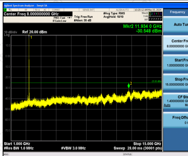
Band41-20MHz-QPSK-41490-1RB#0-Range2:1000~15000MHz
