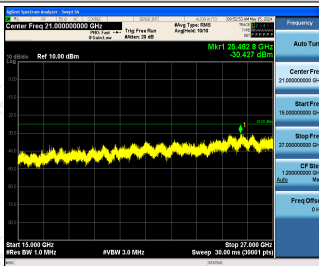
Band41-10MHz-QPSK-39700-1RB#0-Range3:15000~27000MHz
