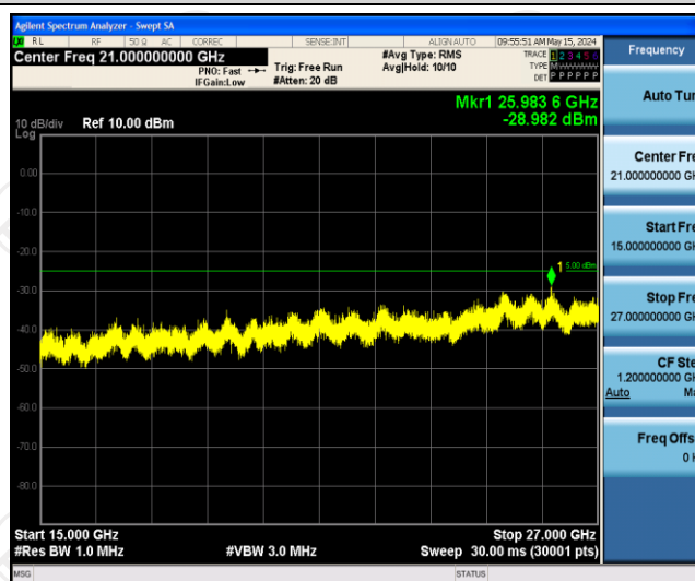
Band41-10MHz-QPSK-41540-1RB#0-Range3:15000~27000MHz
