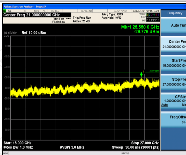
Band41-20MHz-QPSK-39750-1RB#0-Range3:15000~27000MHz
