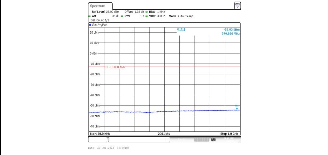
Band2-9538-5-30~1000MHz-PASS
