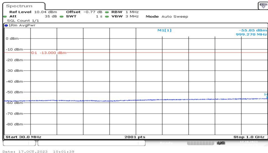
Band2-9538-1-30~1000MHz-PASS
