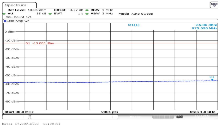
Band2-9400-1-30~1000MHz-PASS
