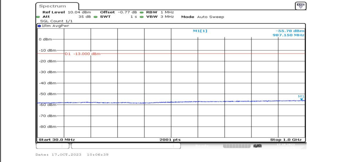
Band2-9538-2-30~1000MHz-PASS
