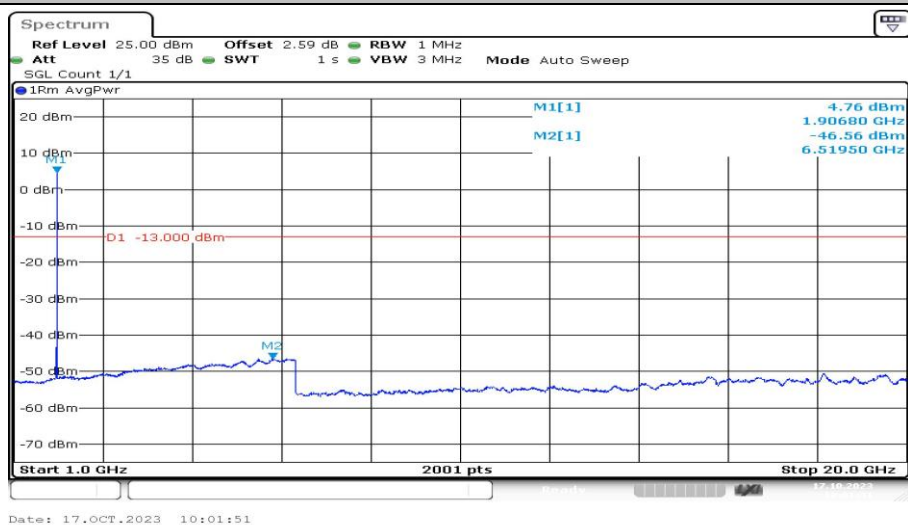
Band2-9538-1-1000~20000MHz-PASS
