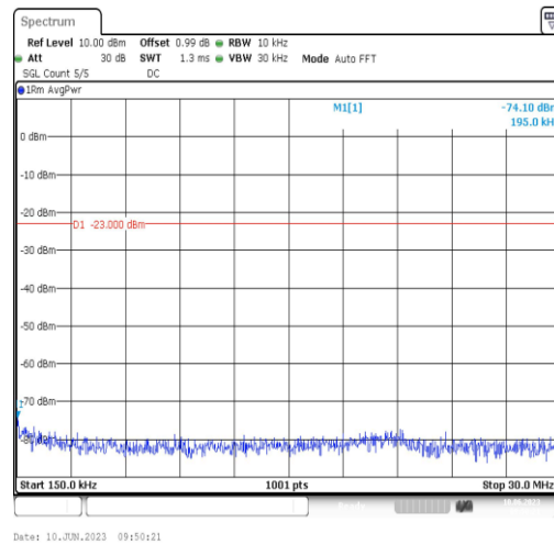
Band71-5MHz-QPSK-133447-1RB#0-Range2:0.15~30MHz
