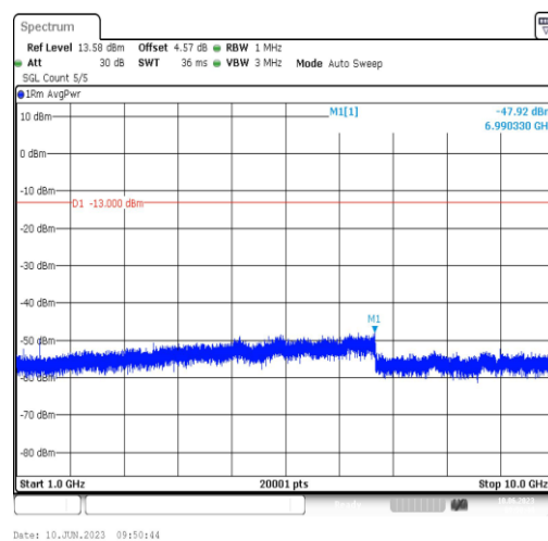
Band71-5MHz-QPSK-133447-1RB#0-Range4:1000~10000MHz
