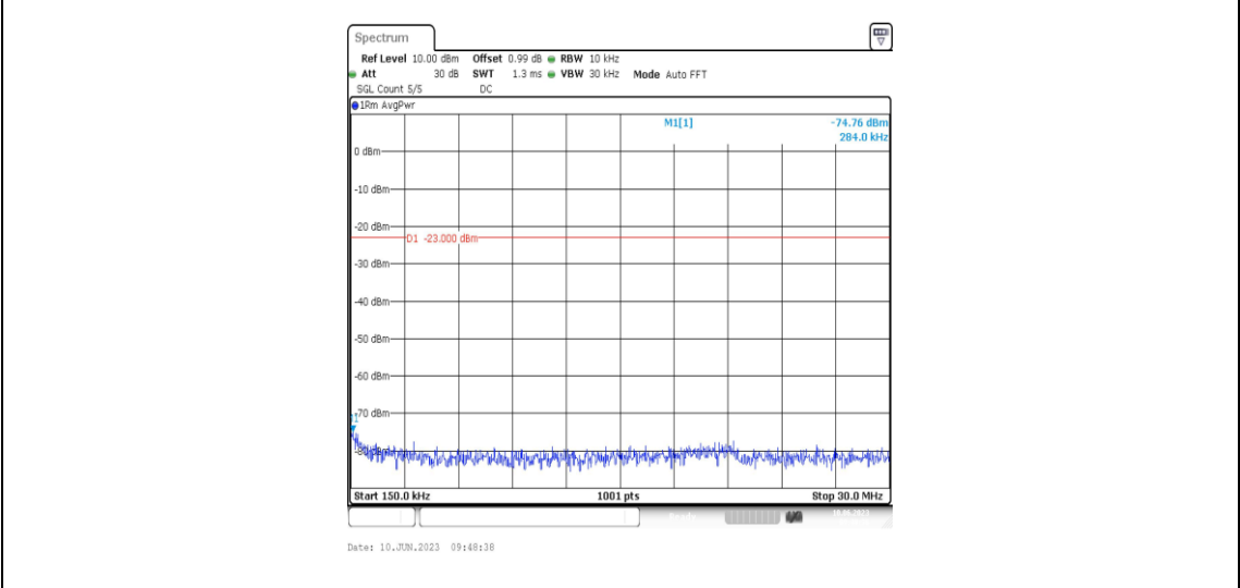
Band71-5MHz-QPSK-133297-1RB#0-Range2:0.15~30MHz
