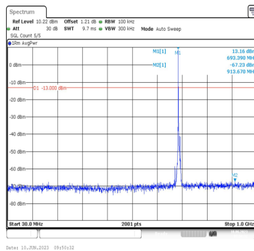
Band71-5MHz-QPSK-133447-1RB#0-Range3:30~1000MHz
