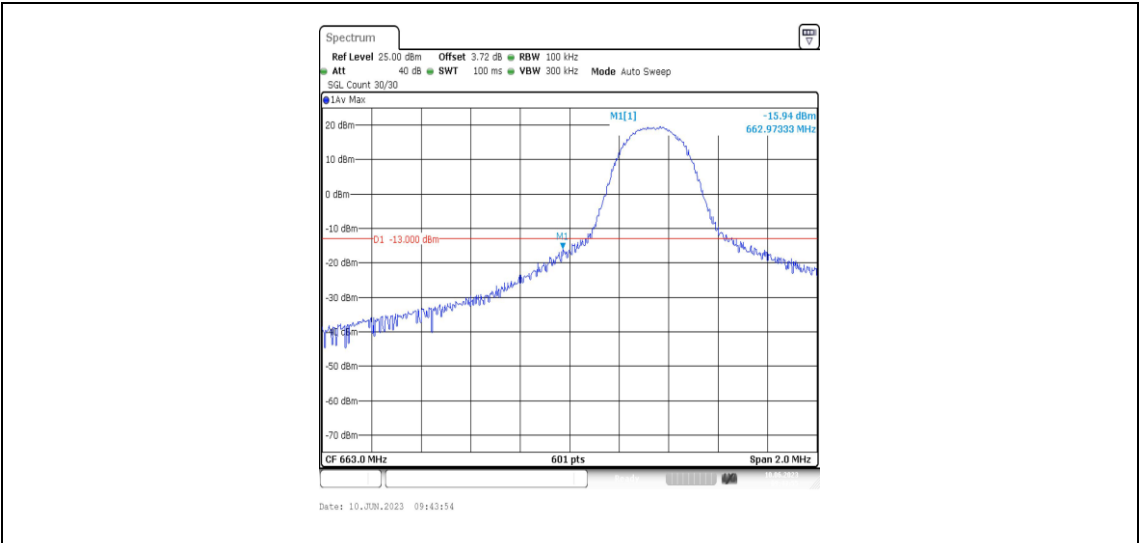
Band71-5MHz-QPSK-133147-1RB#0
