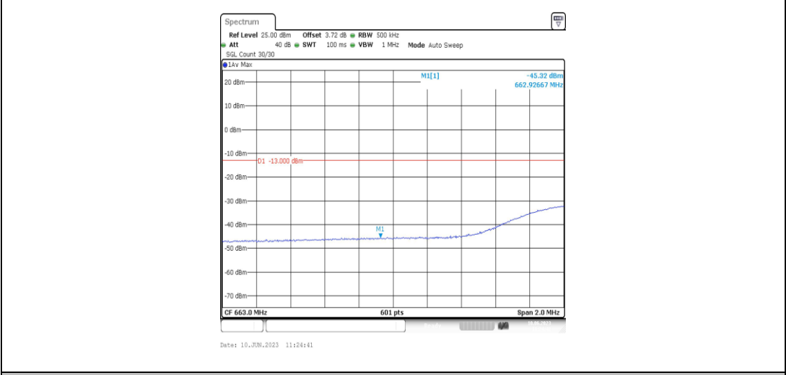
Band71-20MHz-QPSK-133222-1RB#99
