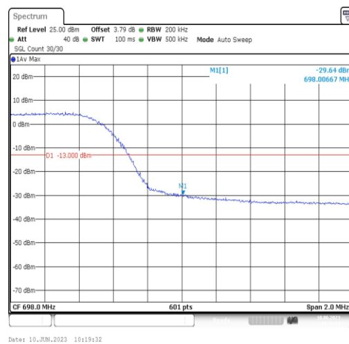
Band71-10MHz-QPSK-133422-50RB#0
