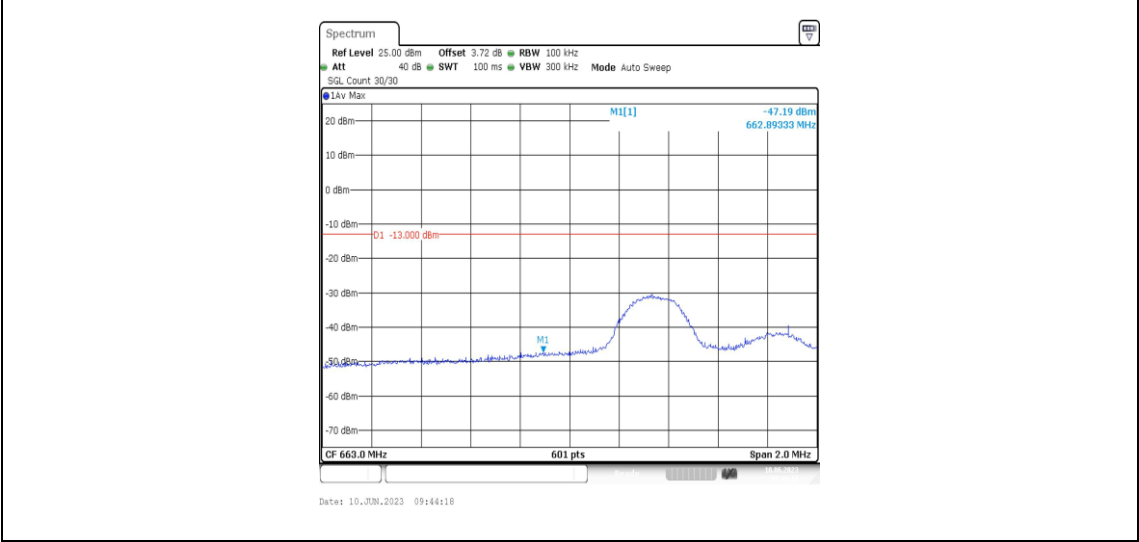
Band71-5MHz-QPSK-133147-1RB#24
