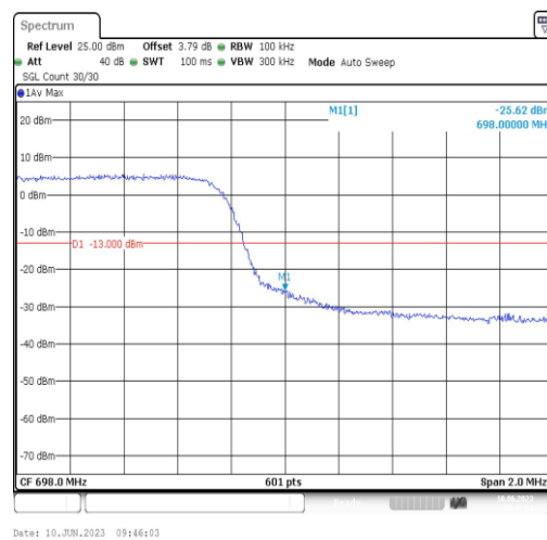
Band71-5MHz-QPSK-133447-25RB#0
