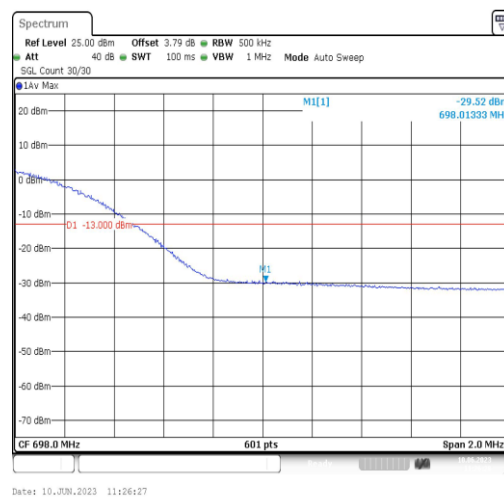
Band71-20MHz-QPSK-133372-100RB#0
