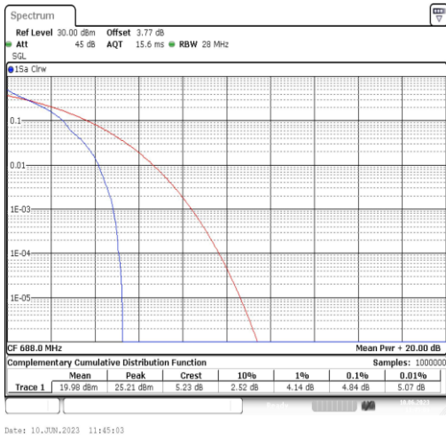
Band71-20MHz-QPSK-133372-1RB#0
