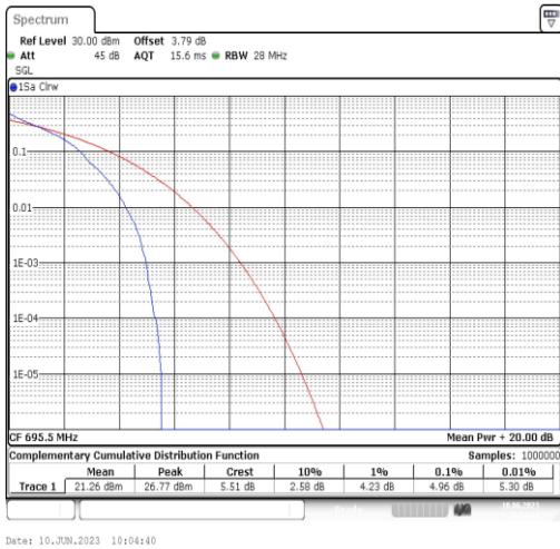
Band71-5MHz-QPSK-133447-1RB#0
