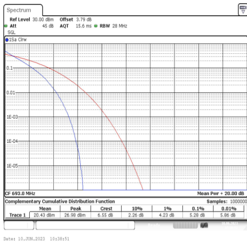
Band71-10MHz-QPSK-133422-50RB#0
