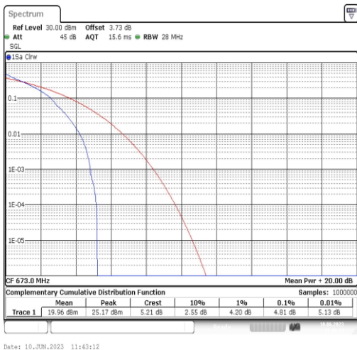
Band71-20MHz-QPSK-133222-1RB#0
