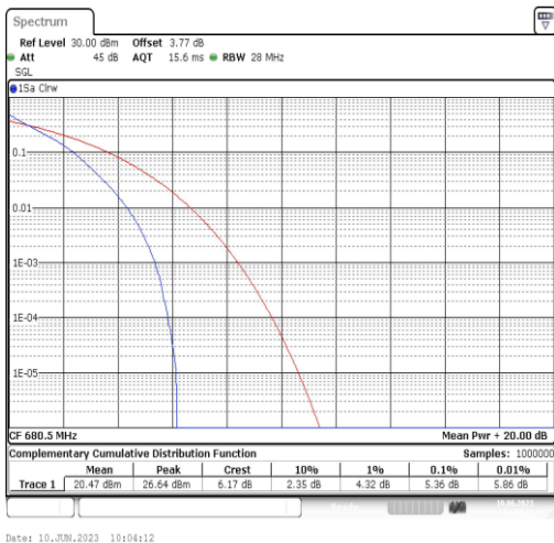
Band71-5MHz-QPSK-133297-25RB#0
