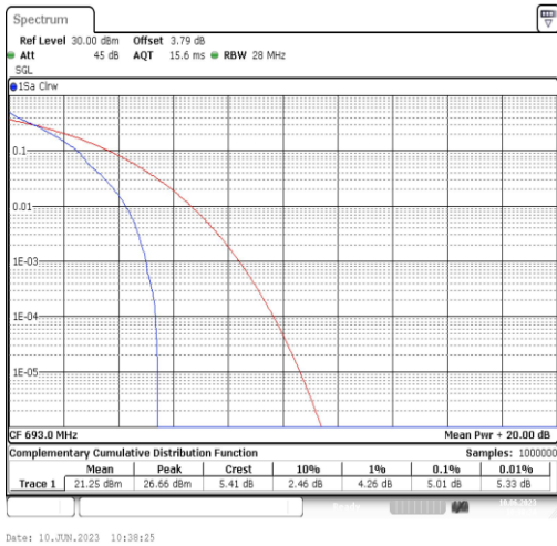
Band71-10MHz-QPSK-133422-1RB#0
