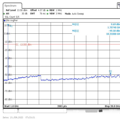
Band66-5MHz-QPSK-131997-1RB#0-Range4:1000~20000MHz
