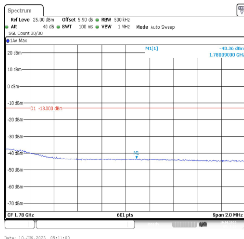
Band66-20MHz-QPSK-132572-1RB#0
