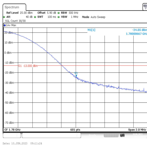
Band66-20MHz-QPSK-132572-1RB#99
