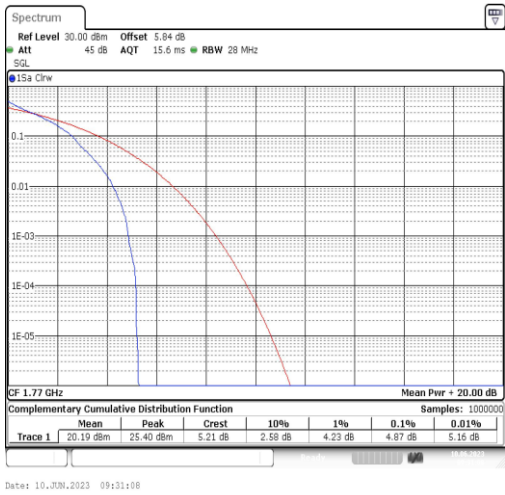
Band66-20MHz-QPSK-132572-1RB#0
