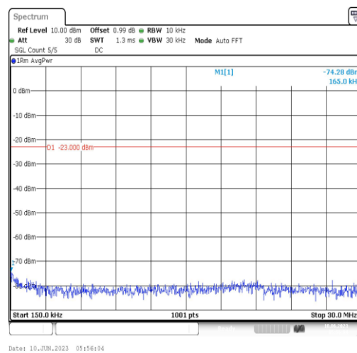
Band12-10MHz-QPSK-23095-1RB#0-Range2:0.15~30MHz
