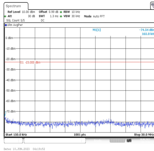
Band12-1.4MHz-QPSK-23173-1RB#0-Range2:0.15~30MHz
