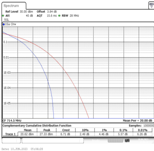
Band12-3MHz-QPSK-23165-15RB#0
