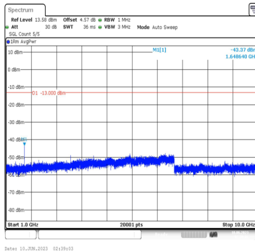
Band5-3MHz-QPSK-20415-1RB#0-Range4:1000~10000MHz
