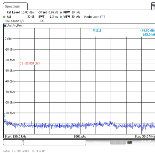
Band5-5MHz-QPSK-20425-1RB#0-Range2:0.15~30MHz
