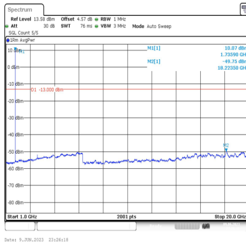
Band4-3MHz-QPSK-20175-1RB#0-Range4:1000~20000MHz
