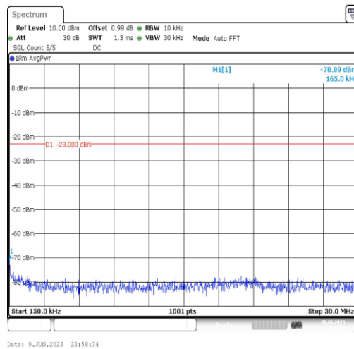
Band4-5MHz-QPSK-20175-1RB#0-Range2:0.15~30MHz
