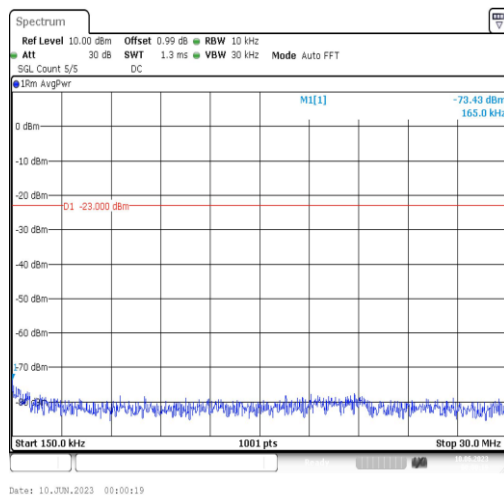
Band4-5MHz-QPSK-20375-1RB#0-Range2:0.15~30MHz
