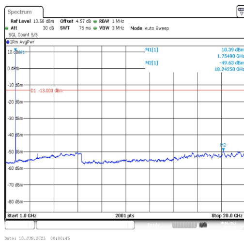
Band4-5MHz-QPSK-20375-1RB#0-Range4:1000~20000MHz
