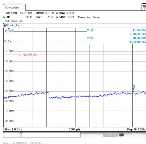
Band4-10MHz-QPSK-20000-1RB#0-Range4:1000~20000MHz
