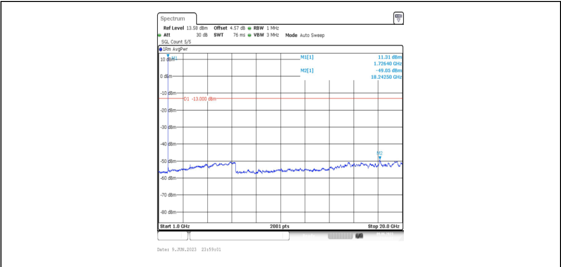
Band4-5MHz-QPSK-20175-1RB#0-Range4:1000~20000MHz
