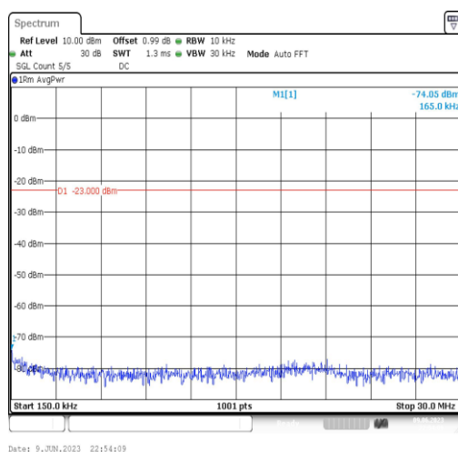
Band4-1.4MHz-QPSK-20175-1RB#0-Range2:0.15~30MHz
