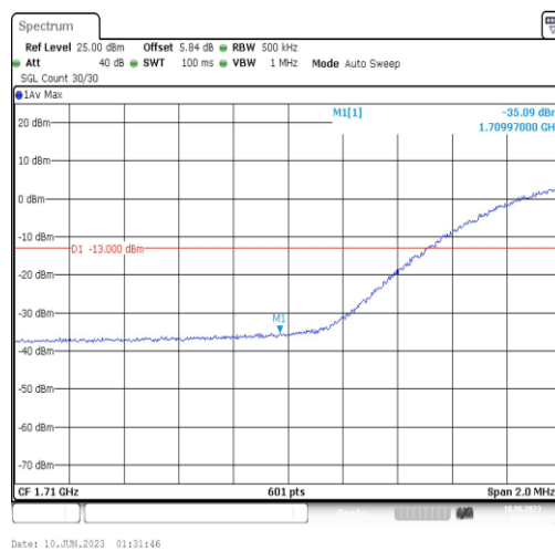
Band4-20MHz-QPSK-20050-100RB#0
