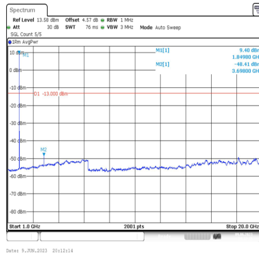
Band2-3MHz-QPSK-18615-1RB#0-Range4:1000~20000MHz
