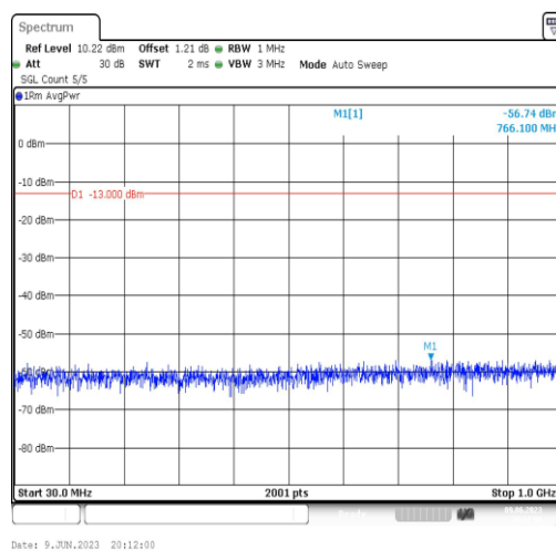
Band2-3MHz-QPSK-18615-1RB#0-Range3:30~1000MHz
