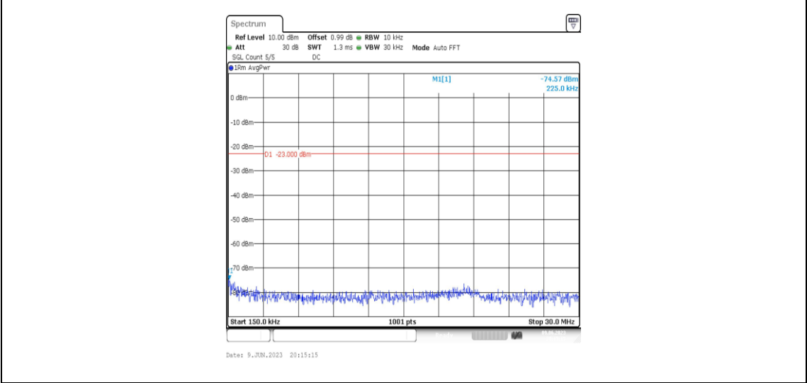
Band2-3MHz-QPSK-19185-1RB#0-Range2:0.15~30MHz
