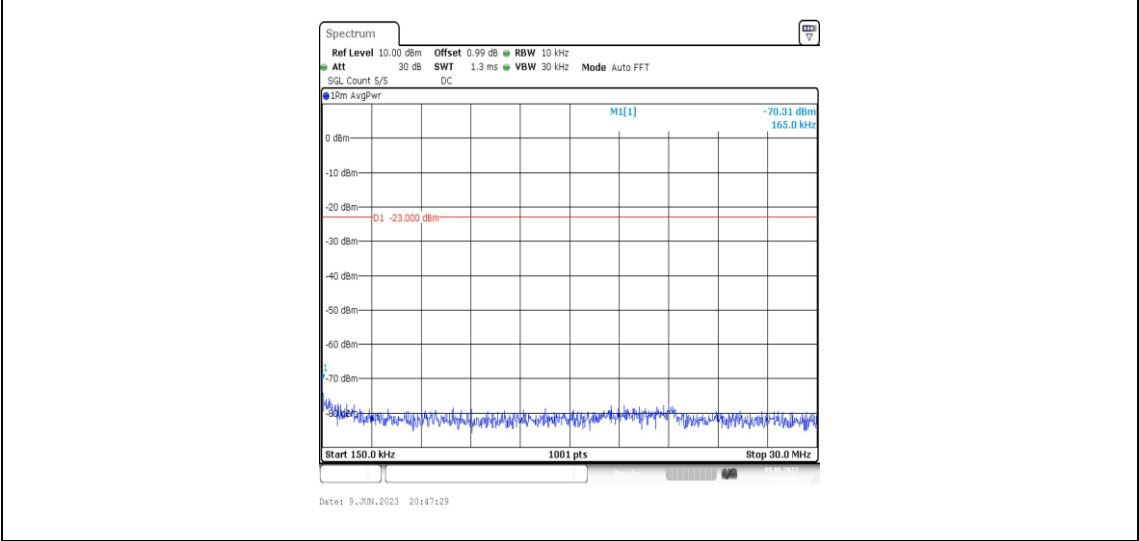
Band2-5MHz-QPSK-19175-1RB#0-Range2:0.15~30MHz
