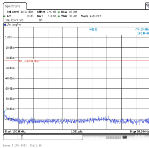
Band2-3MHz-QPSK-18615-1RB#0-Range2:0.15~30MHz
