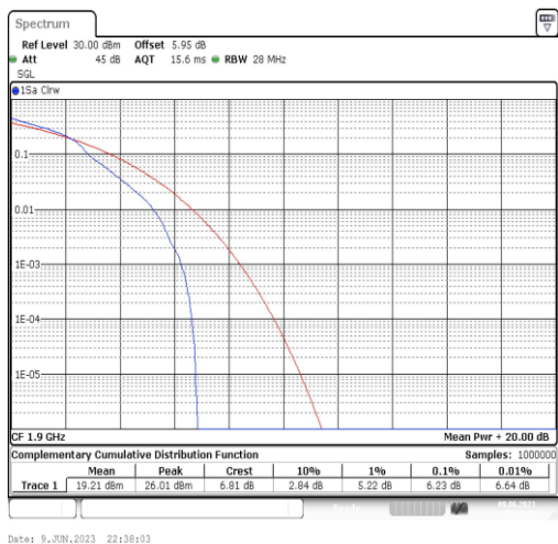
Band2-20MHz-16QAM-19100-1RB#0
