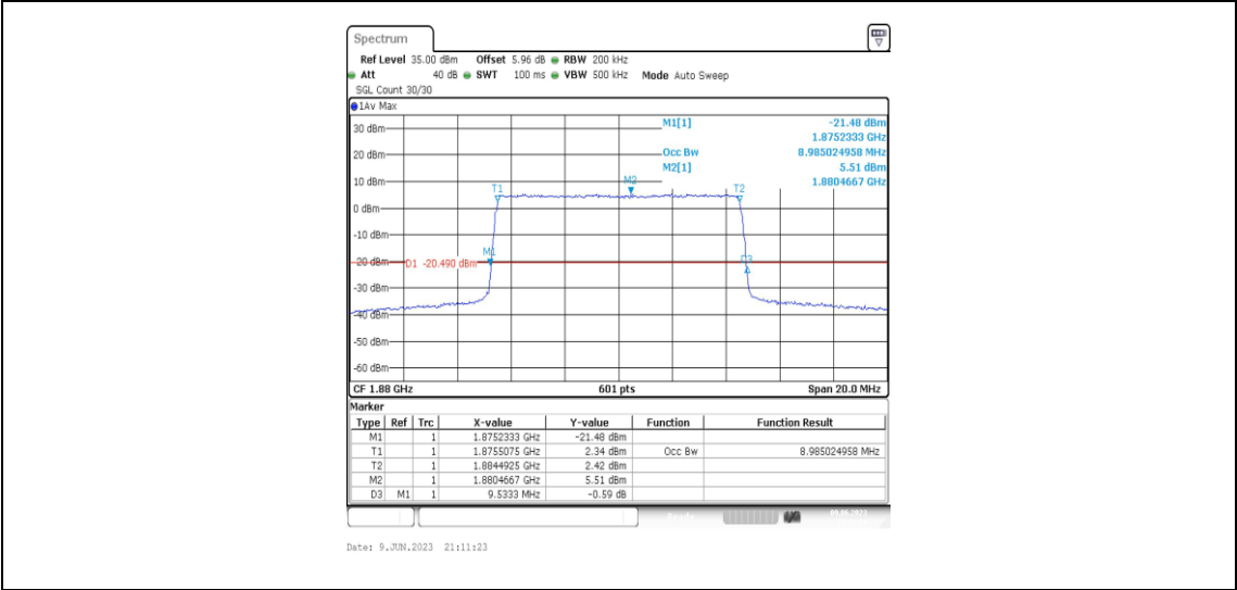
Band2-10MHz-QPSK-18900-50RB#0-8.985
