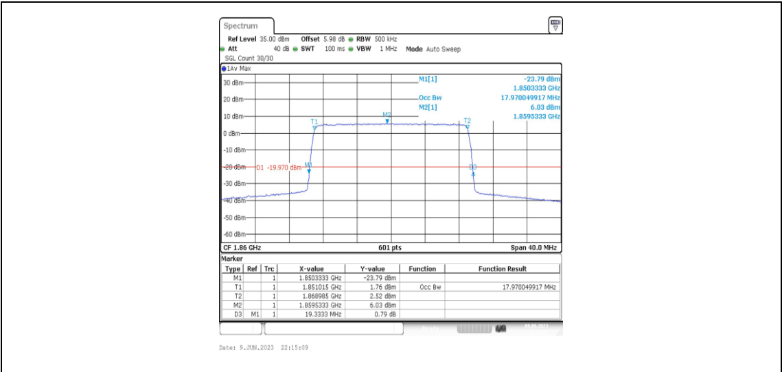
Band2-20MHz-QPSK-18700-100RB#0-17.97
