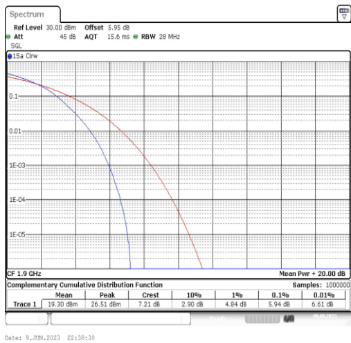
Band2-20MHz-16QAM-19100-100RB#0
