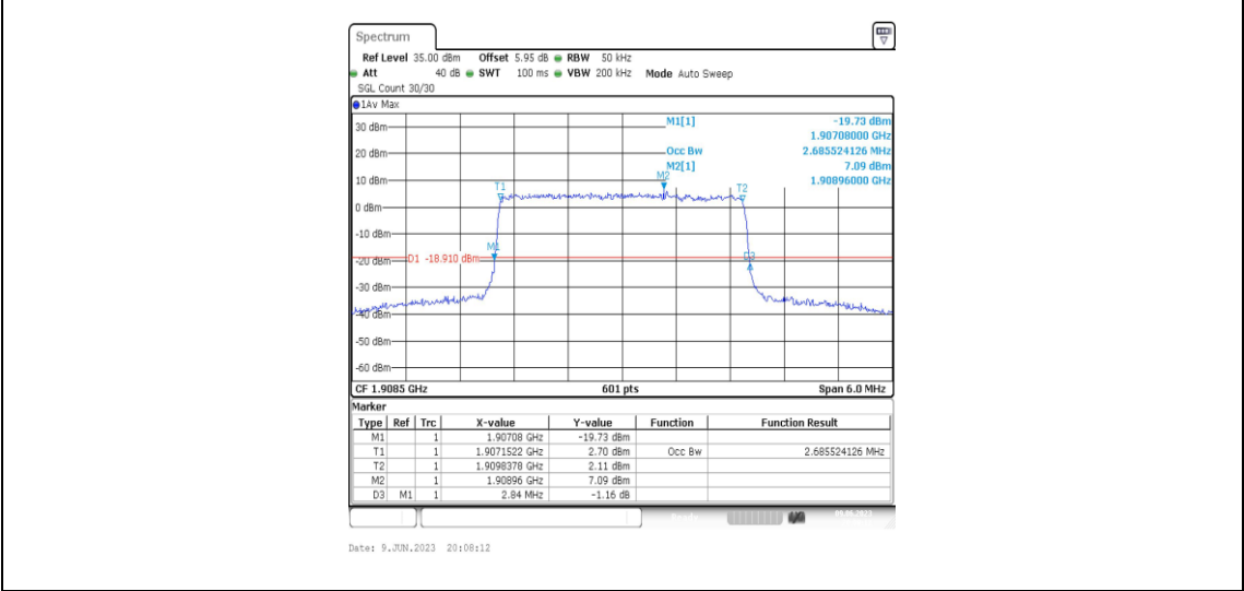
Band2-3MHz-16QAM-19185-15RB#0-2.686
