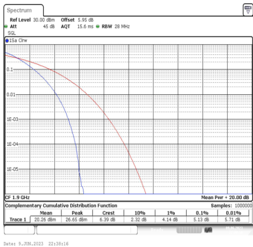
Band2-20MHz-QPSK-19100-100RB#0
