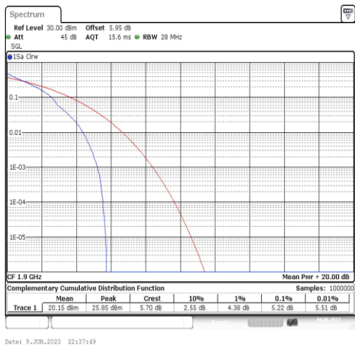
Band2-20MHz-QPSK-19100-1RB#0
