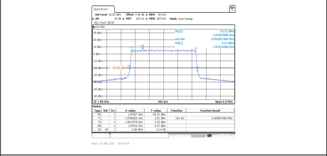
Band2-3MHz-QPSK-18900-15RB#0-2.696
