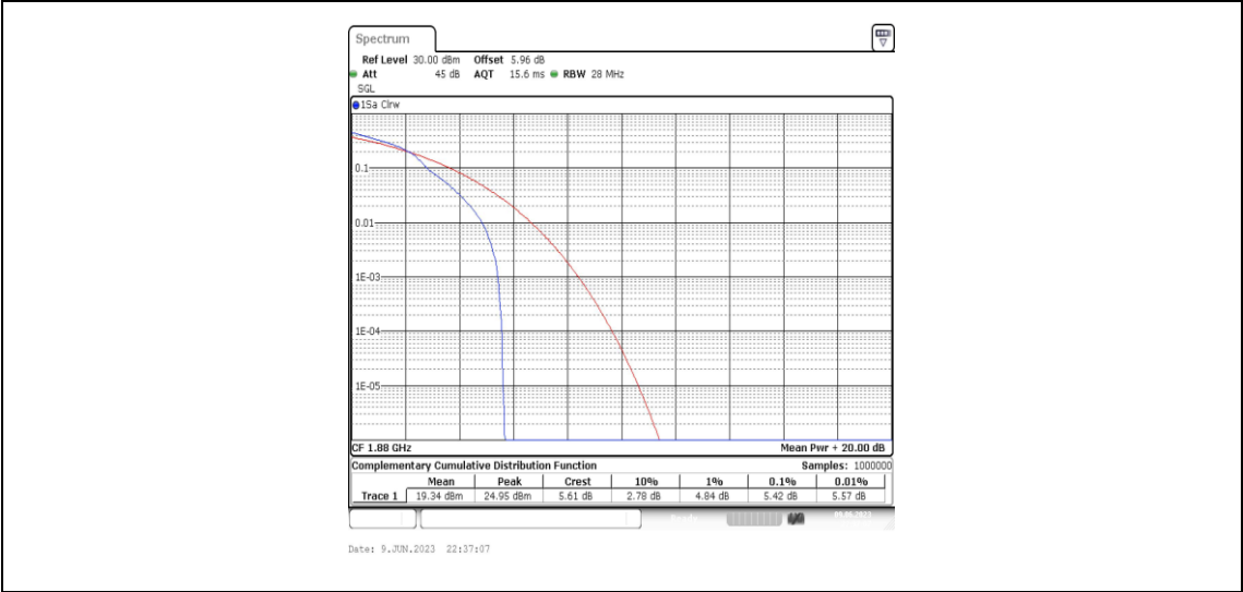
Band2-20MHz-16QAM-18900-1RB#0
