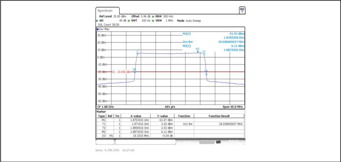
Band2-20MHz-QPSK-18900-100RB#0-18.037
