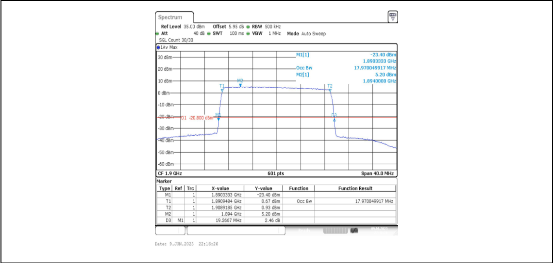
Band2-20MHz-16QAM-19100-100RB#0-17.97
