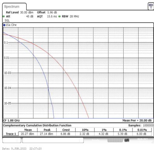
Band2-20MHz-QPSK-18900-100RB#0
