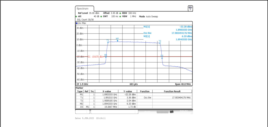
Band2-20MHz-QPSK-19100-100RB#0-17.903
