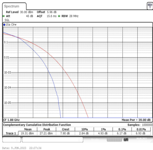
Band2-20MHz-16QAM-18900-100RB#0
