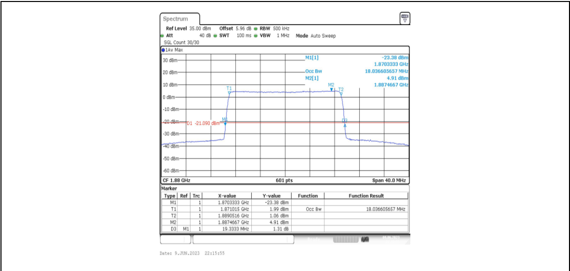
Band2-20MHz-16QAM-18900-100RB#0-18.037
