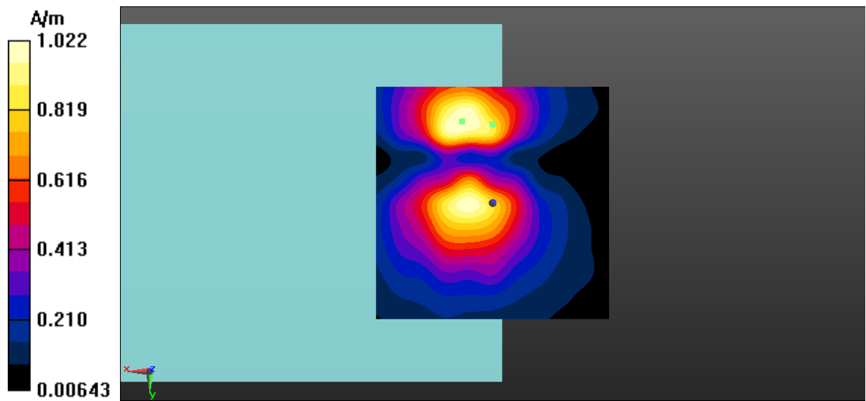
Fig A.17 T-Coil EDGE 850-Y
