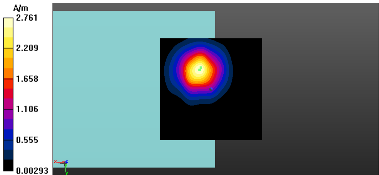
Fig A.17 T-Coil EDGE 850-Z
