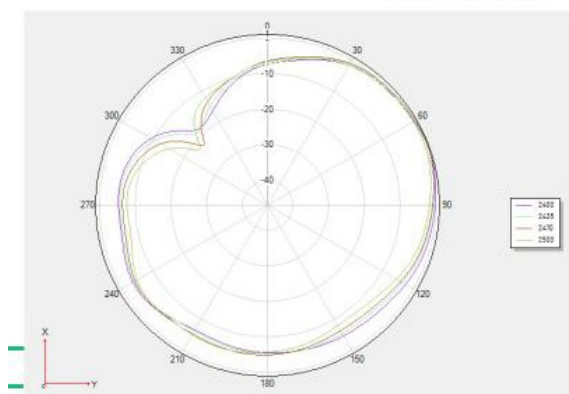
Theta 90 2D图
