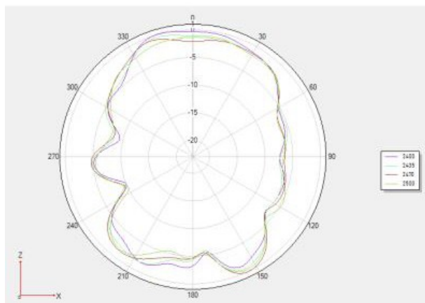
Phi 0 2D图
