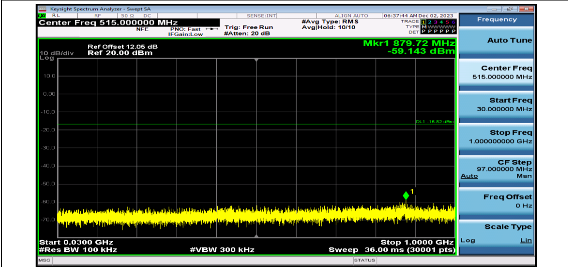
DH5-Ant1-2441-30~1000
