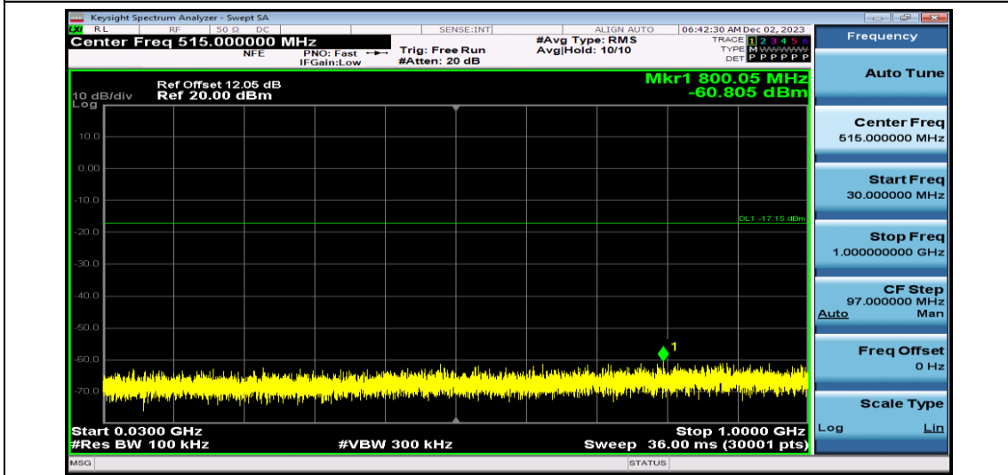
2DH5-Ant1-2402-30~1000
