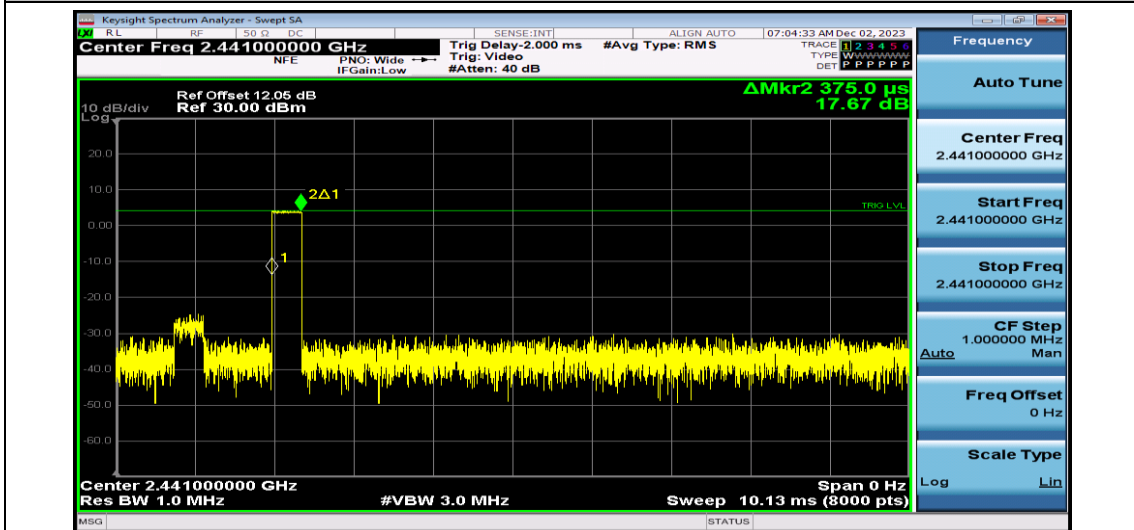
DH1-Ant1-Hop
