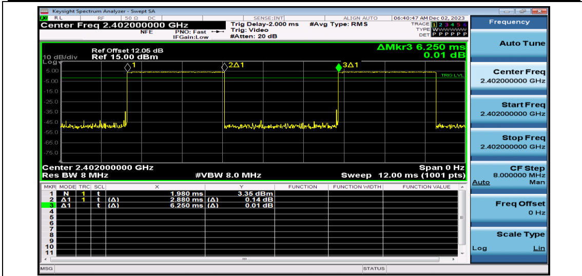
NTNV-2DH5-Ant1-2402
