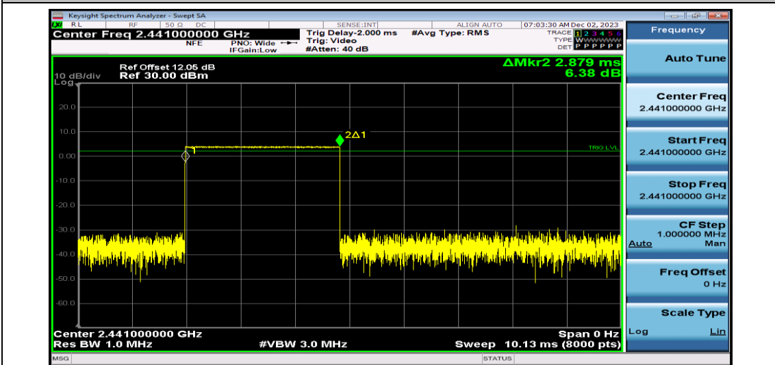
DH5-Ant1-Hop
