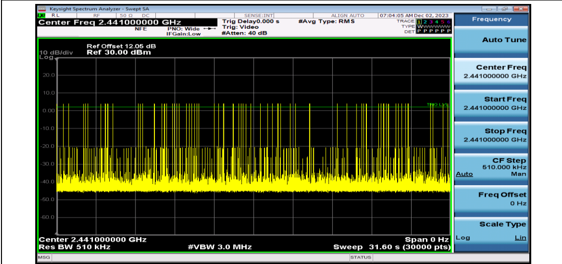
DH5-Ant1-Hop
