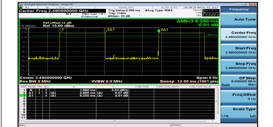
NTNV-DH5-Ant1-2480
