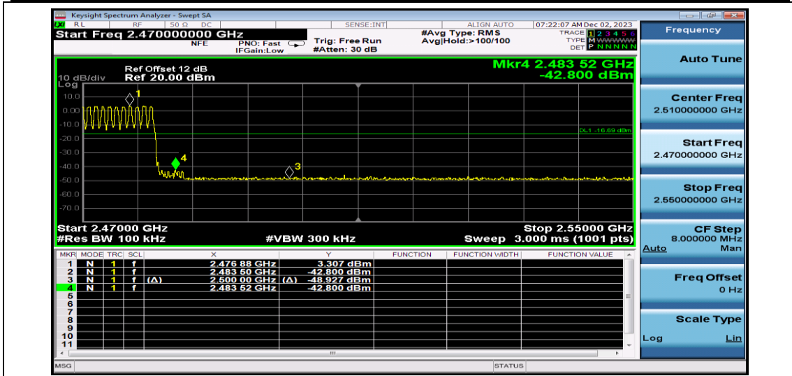
DH5-Ant1-Hop_2480
