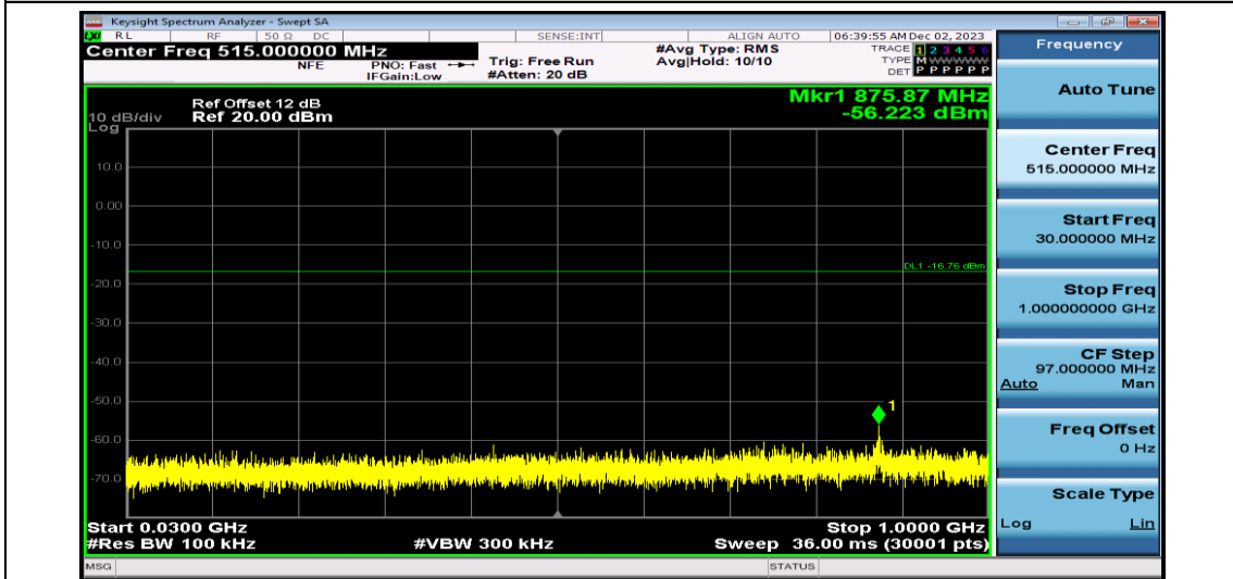
DH5-Ant1-2480-30~1000
