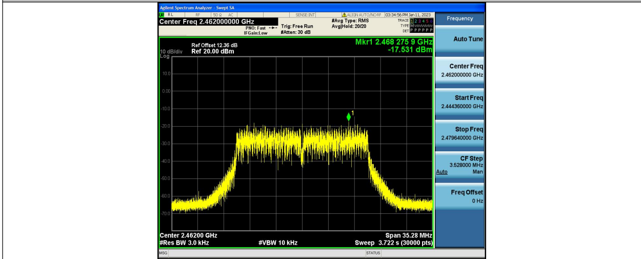
11N20SISO-Ant1-2462--17.53-0.00-0.00-0.00
