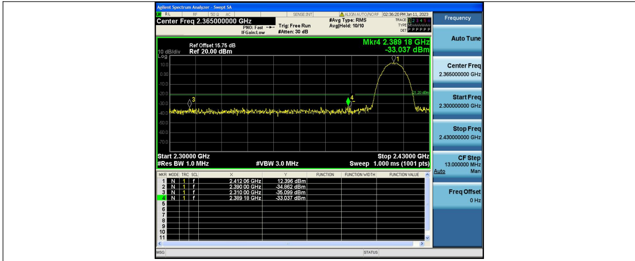
11B-Ant1-Low-2412-AV-2390.000
