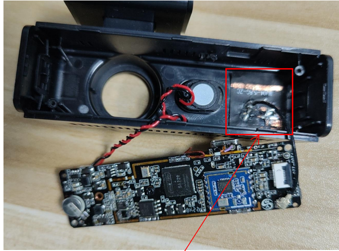
Antenna
