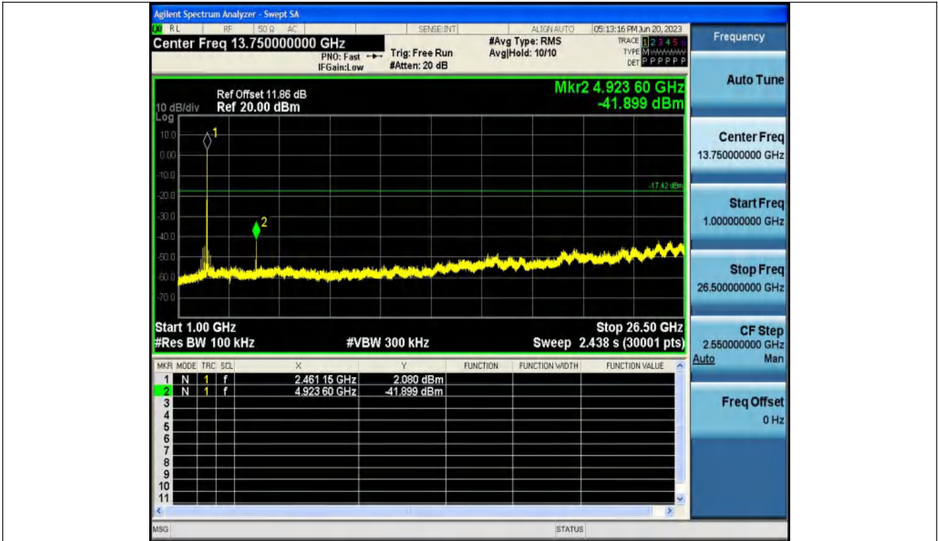
11B-Ant1-2462-1000~26500
