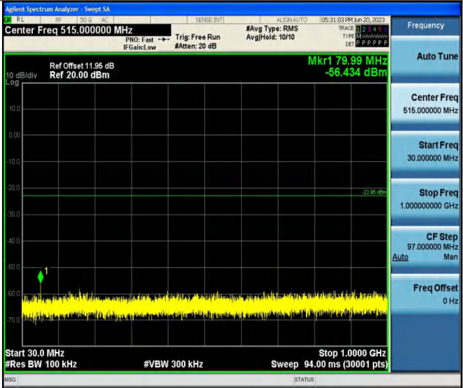
11G-Ant1-2412-30~1000
