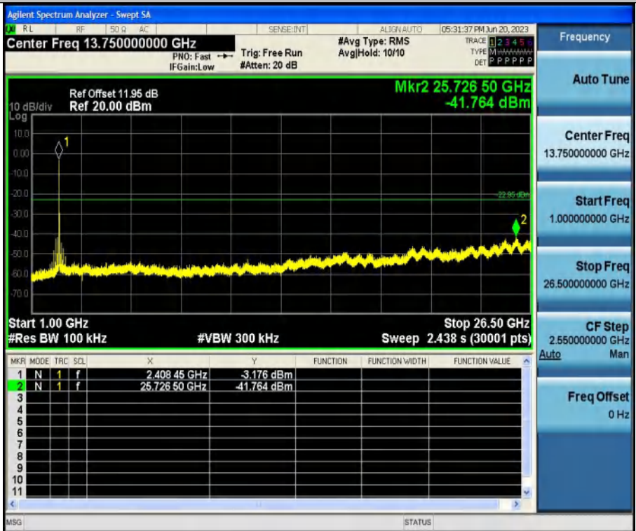
11G-Ant1-2412-1000~26500
