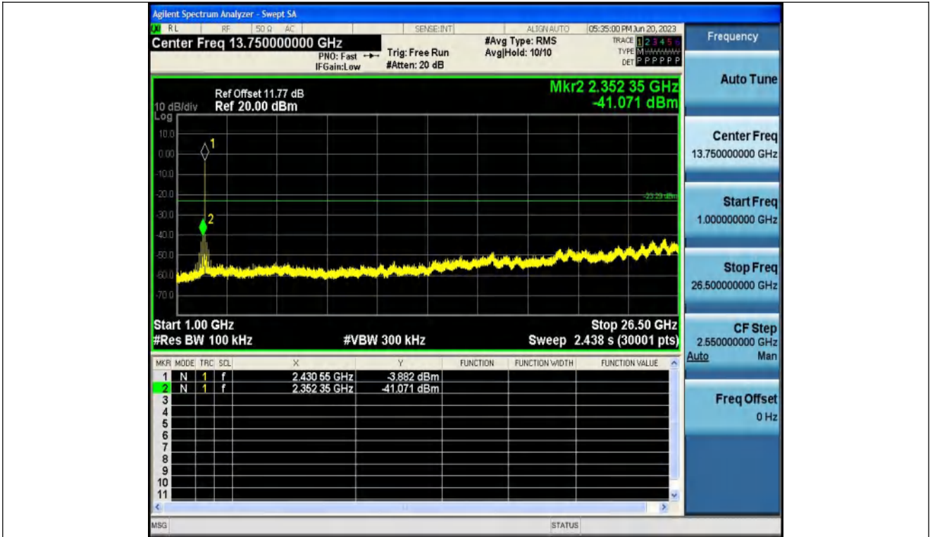
11G-Ant1-2437-1000~26500
