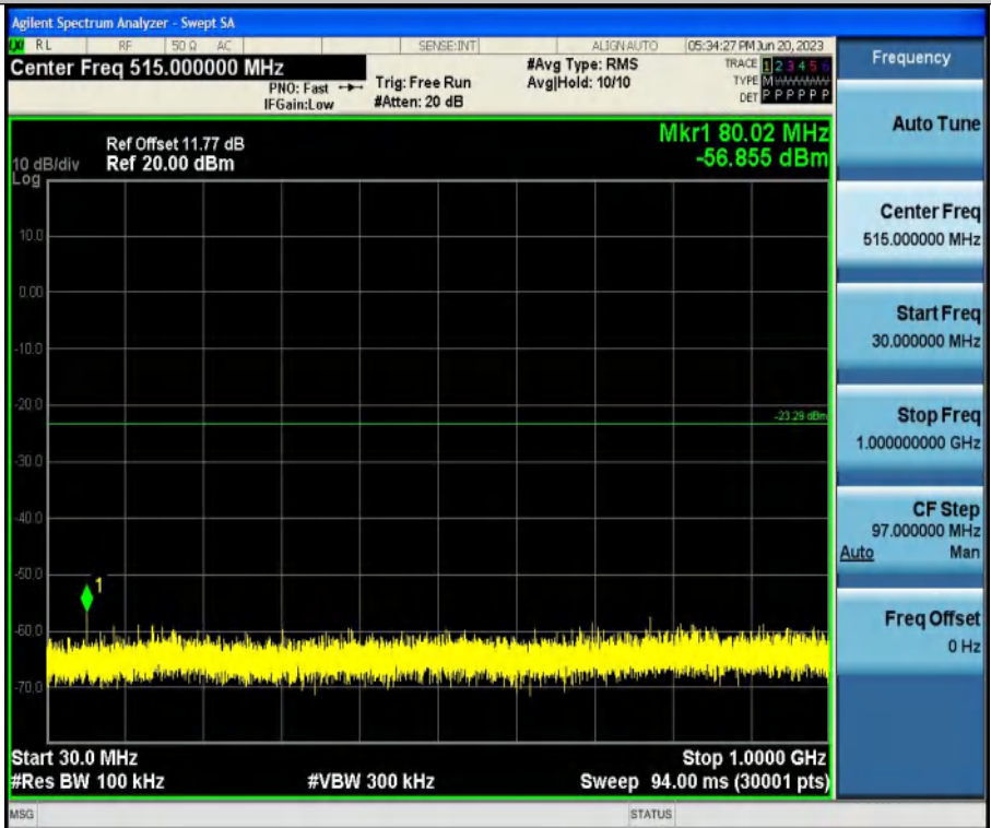
11G-Ant1-2437-30~1000
