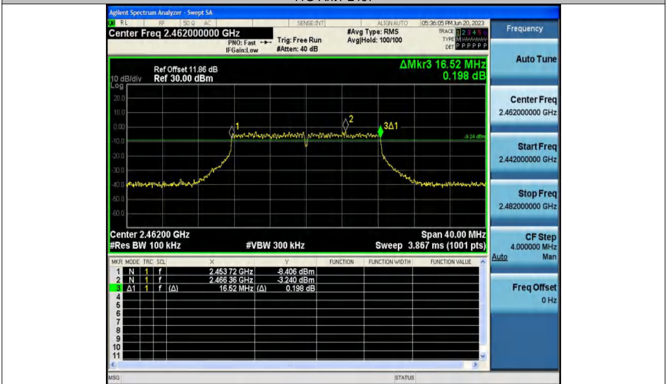
11G-Ant1-2462
