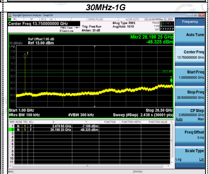
1G-26.5G
