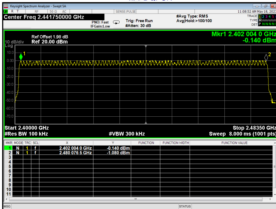
\pi/4 -DQPSK
