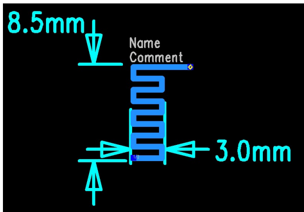
Antenna
