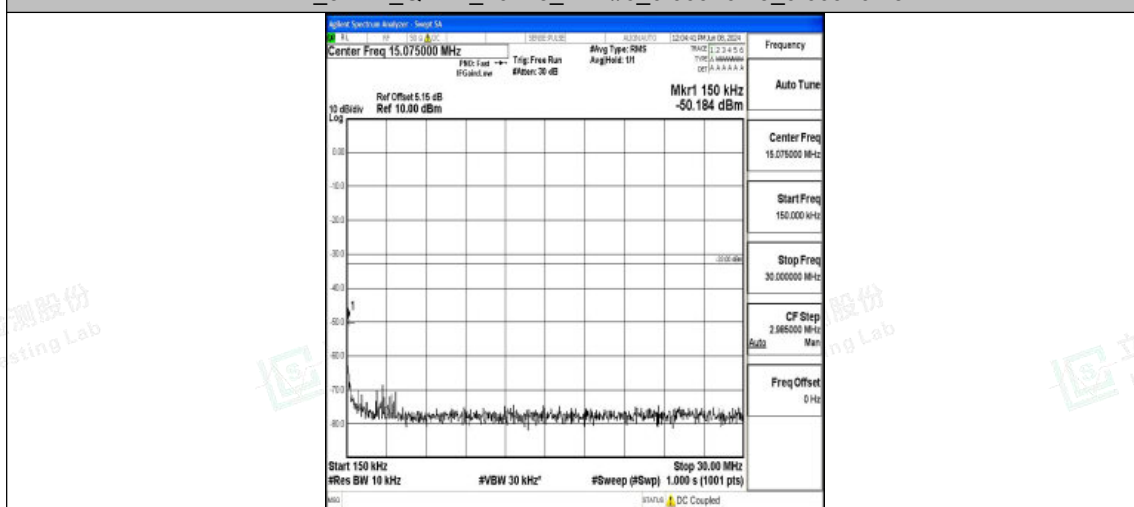
Band4 5MHz QPSK 20175 1RB#0 0.15~30 0.15~30
