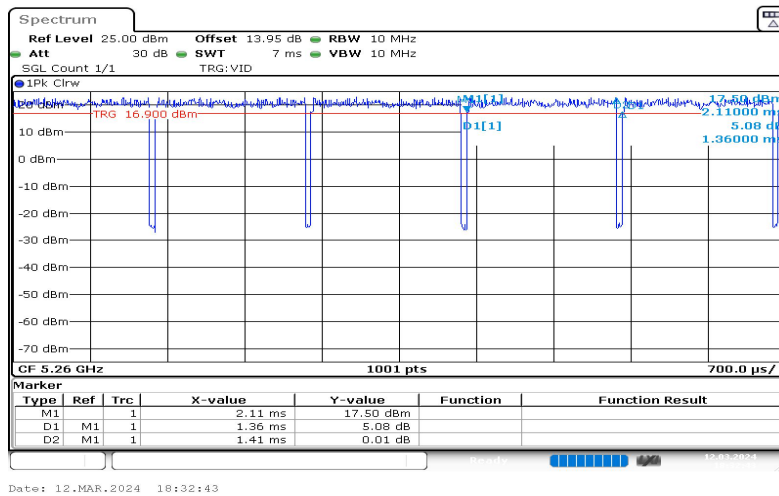
NTNV-11A-Ant1-5260-1.36-1.41
