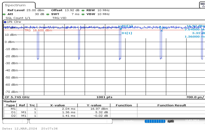
NTNV-11A-Ant1-5745-1.36-1.41
