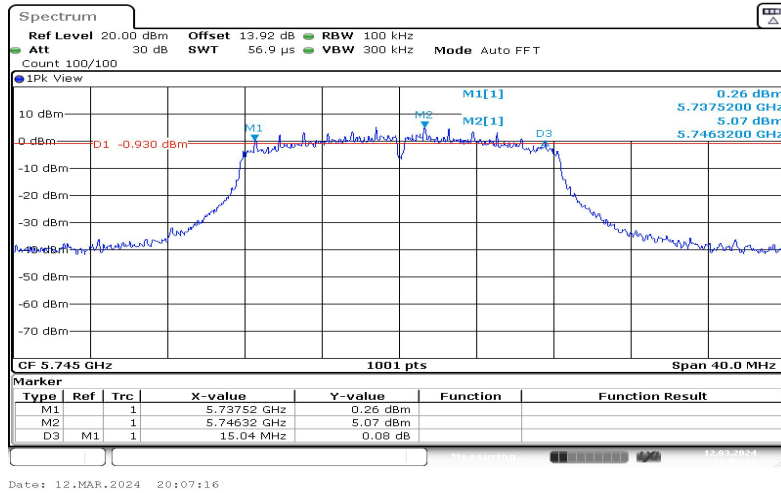
11A-Ant1-5745
